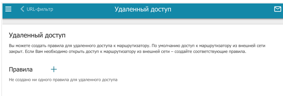
Рисунок 197. Страница Межсетевой экран / Удаленный доступ .
