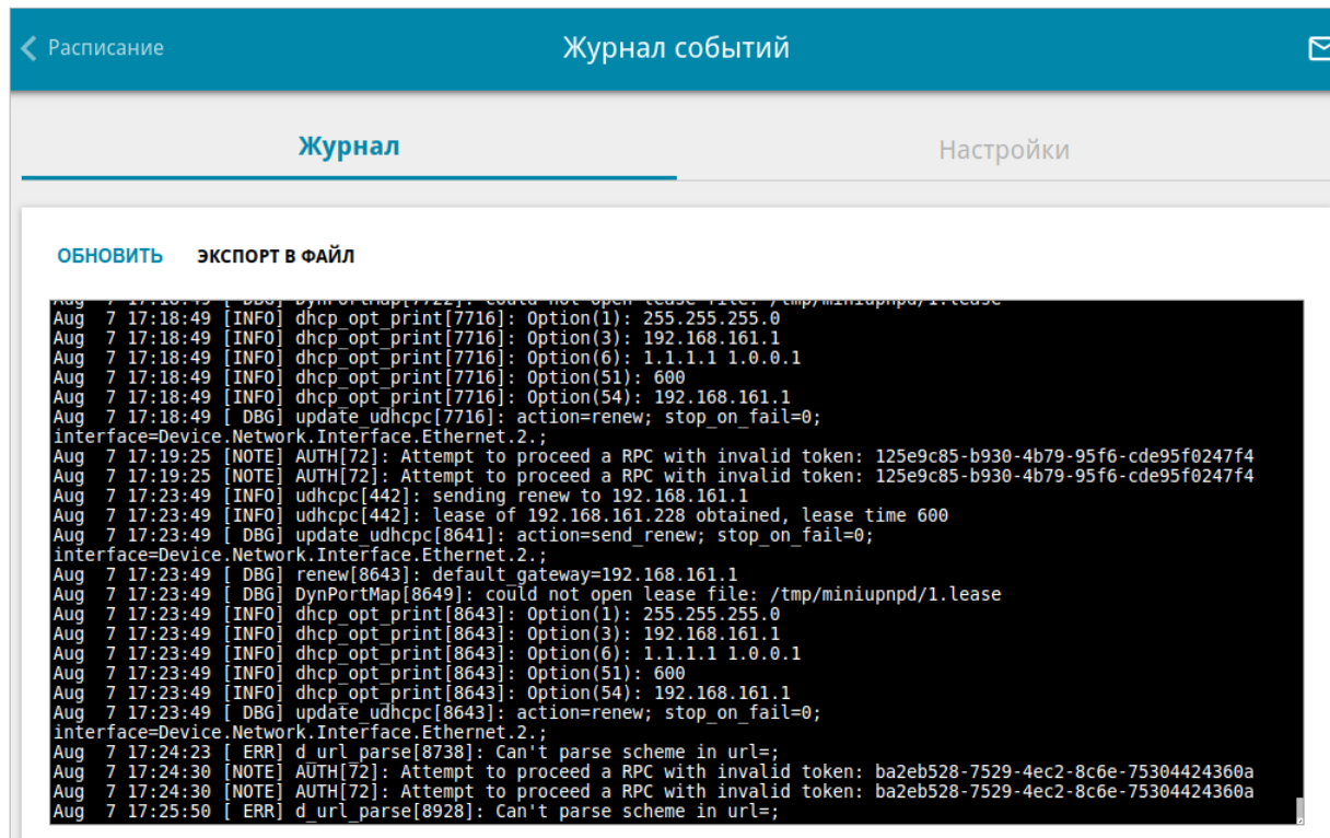
Рисунок 207. Страница Система / Журнал событий. Вкладка Журнал.
