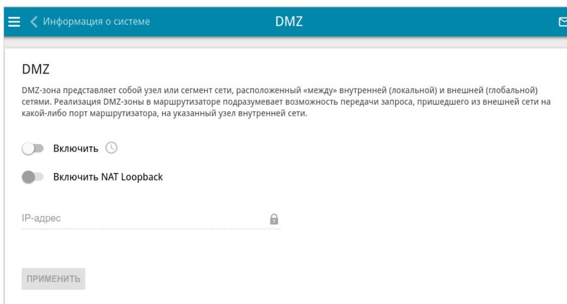
Рисунок 192. Страница Межсетевой экран / DMZ .
