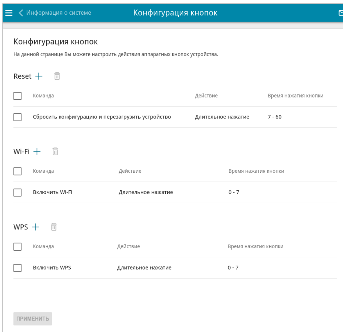
Рисунок 200. Страница Система / Конфигурация кнопок .
