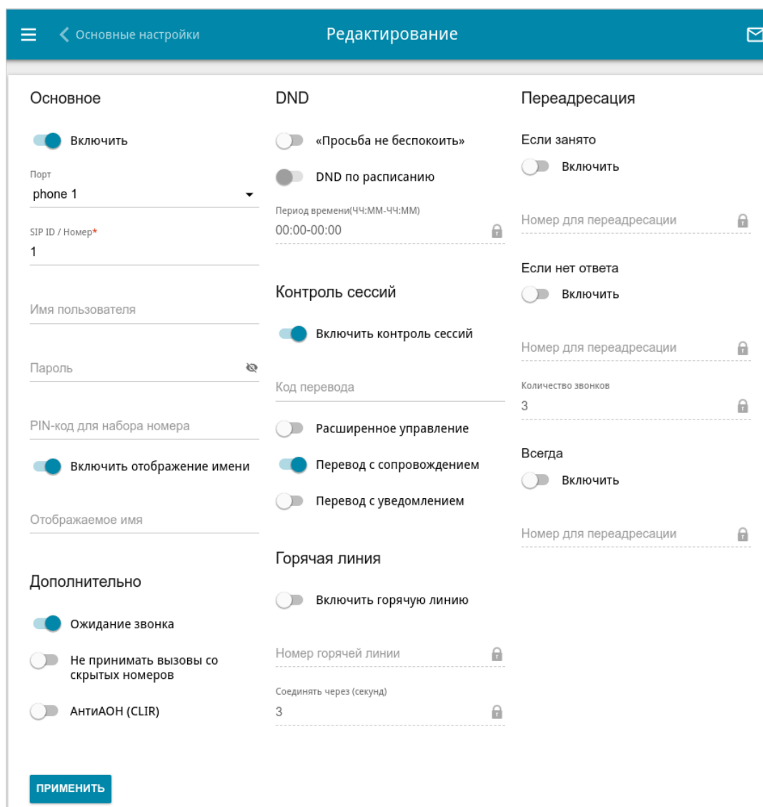
Рисунок 173. Страница изменения параметров SIP-линии.
