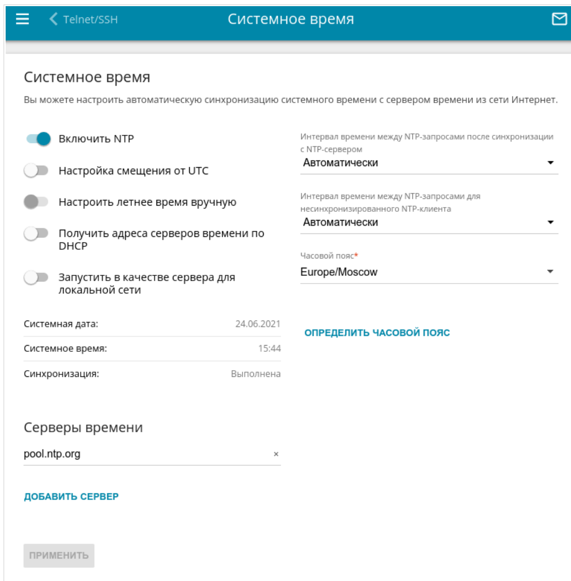
Рисунок 213. Страница Система / Системное время .
