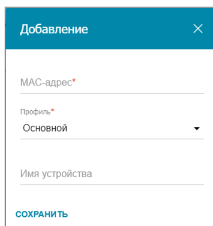
Рисунок 217. Страница SkyDNS / Устройства и правила . Окно добавления правила.
