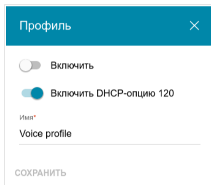
Рисунок 163. Окно добавления профиля.
