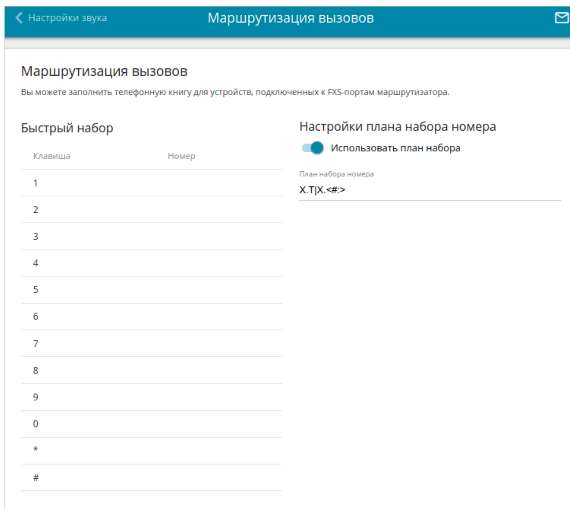
Рисунок 183. Страница VoIP / Имя профиля / Маршрутизация вызовов .
