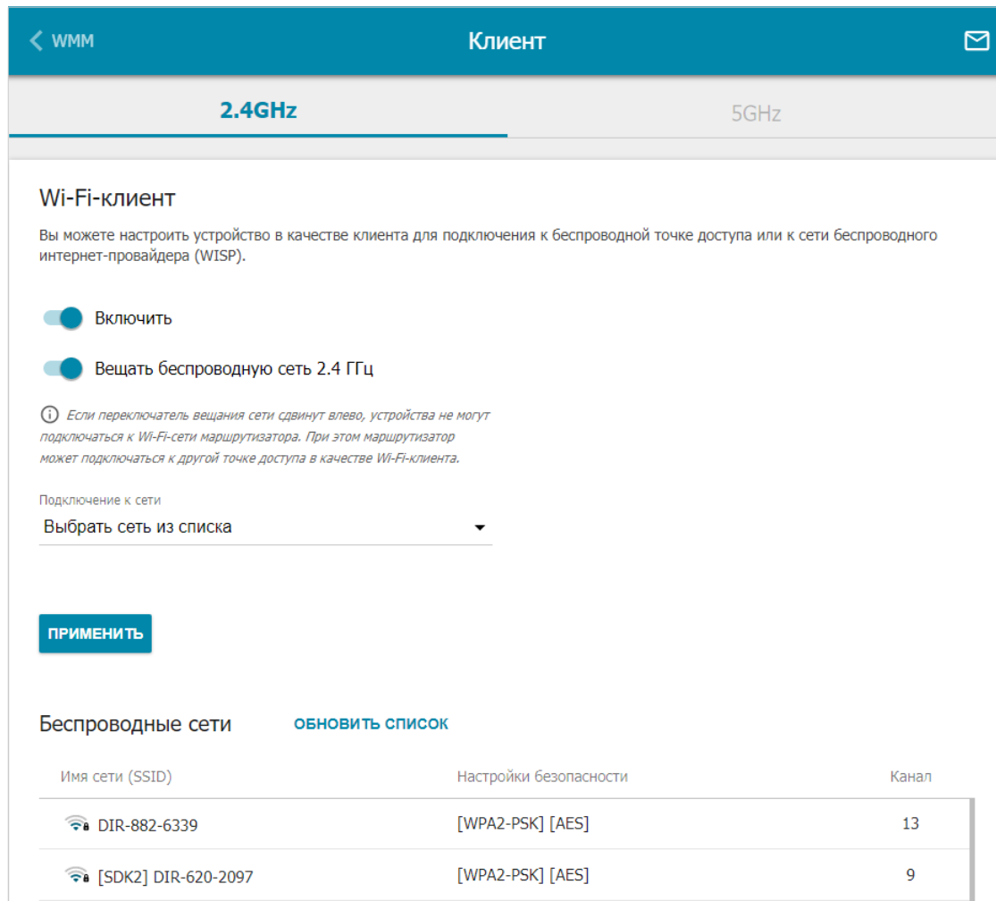
Рисунок 130. Страница для настройки маршрутизатора в качестве клиента.
