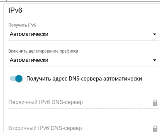
Рисунок 85. Страница добавления соединения типа PPPoE IPv6. Раздел IPv6.
