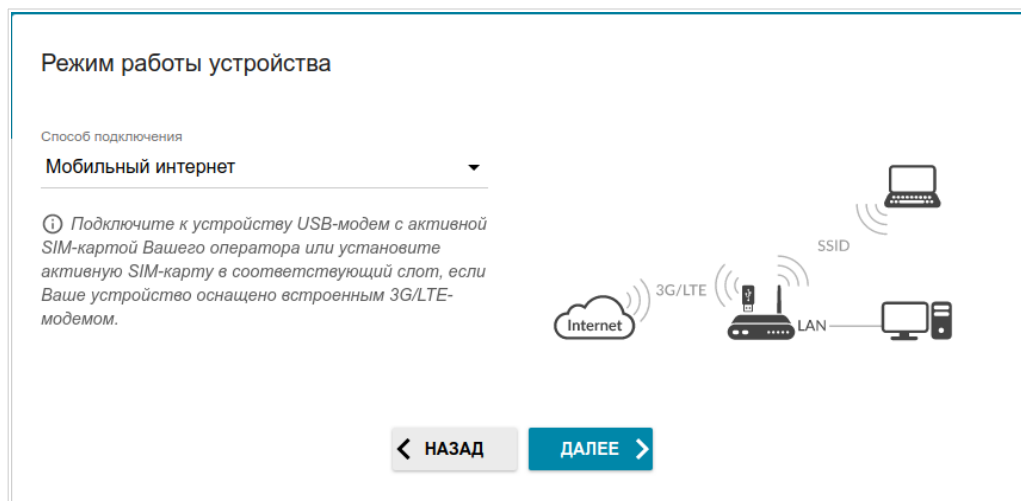
Рисунок 36. Выбор режима работы устройства. Режим Мобильный интернет .
