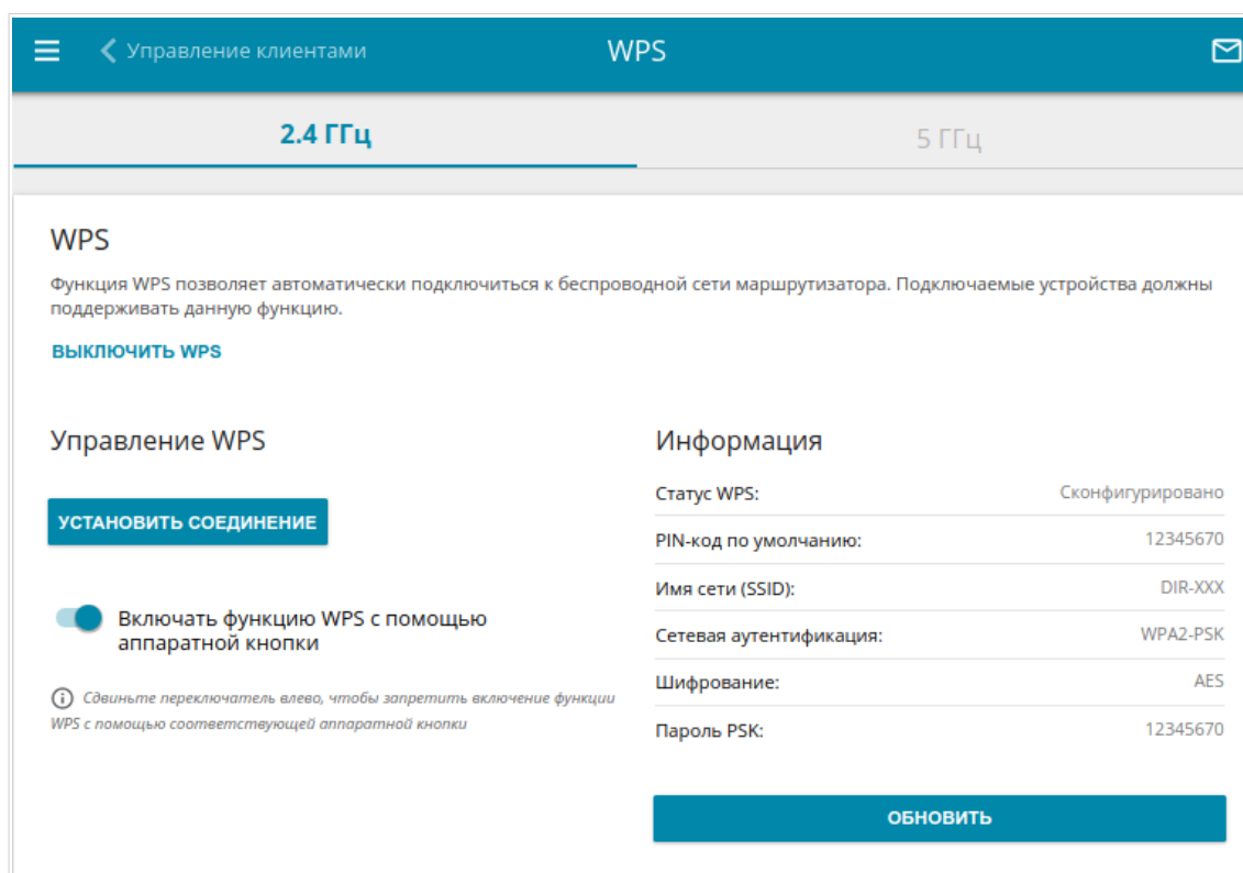
Рисунок 103. Страница для настройки функции WPS.
