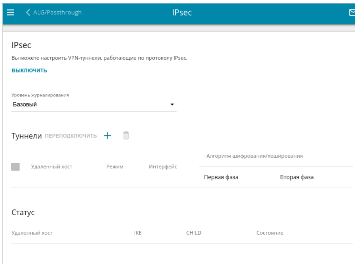
Рисунок 124. Страница Дополнительно / IPsec .
