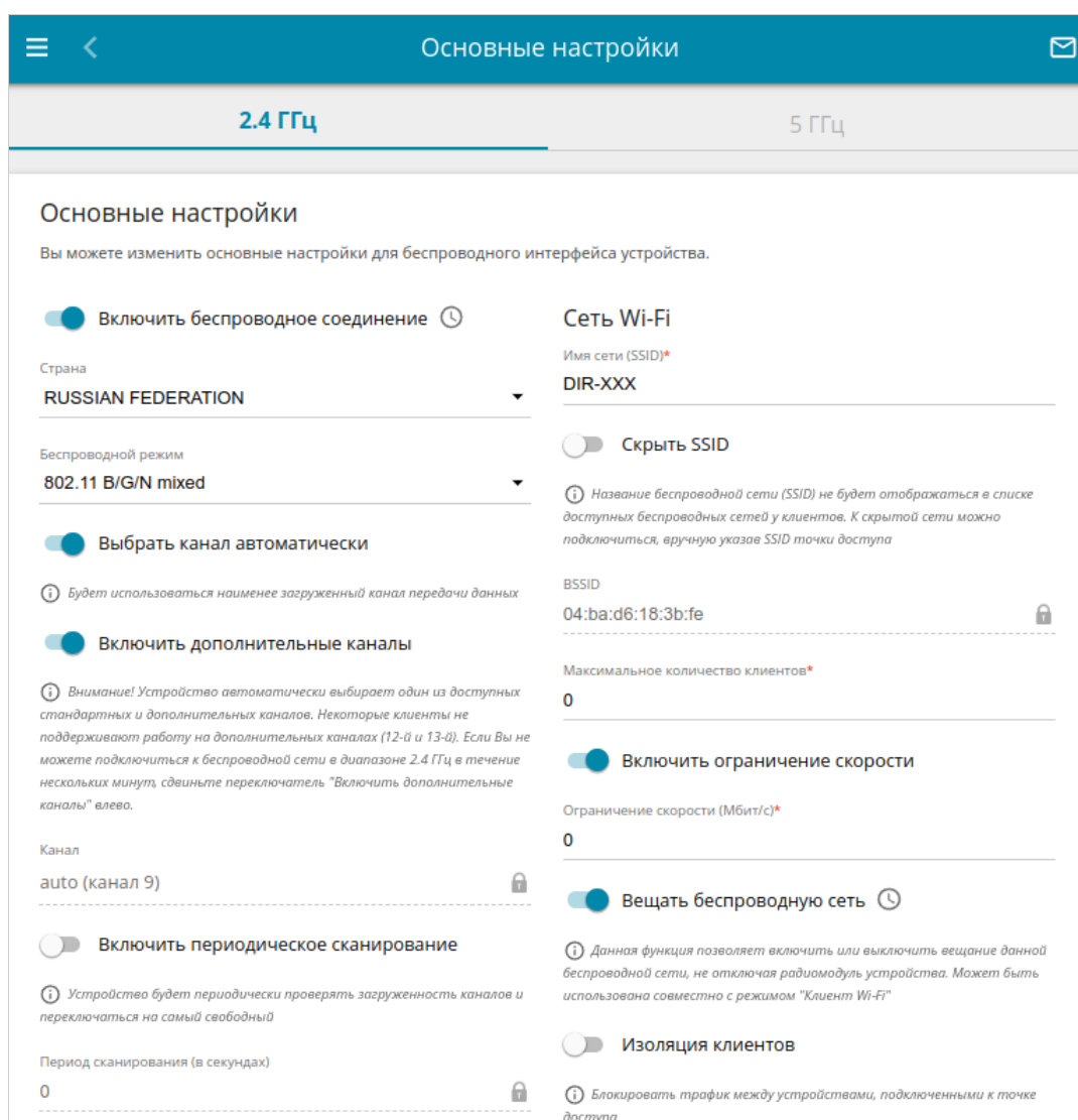
Рисунок 96. Основные настройки беспроводной локальной сети в диапазоне 2,4 ГГц.
