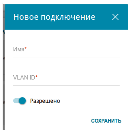
Рисунок 48. Добавление подключения.
