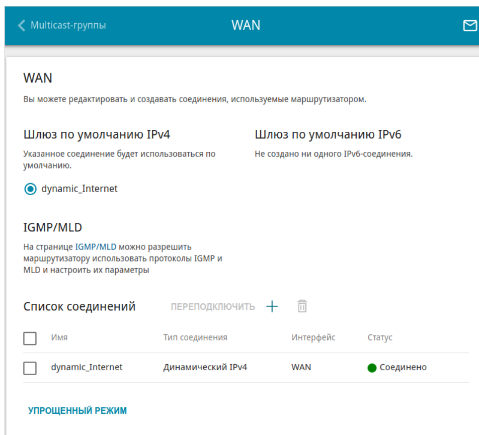
Рисунок 66. Страница Настройка соединений / WAN . Расширенный режим.
