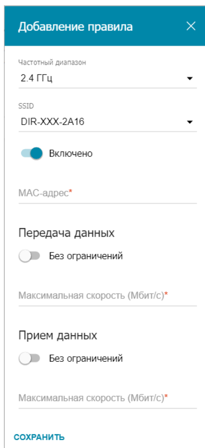
Рисунок 116. Окно для настройки ограничения скорости.
