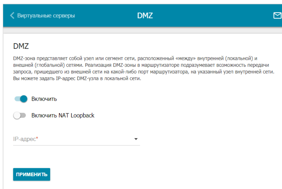
Рисунок 165. Страница Межсетевой экран / DMZ .
