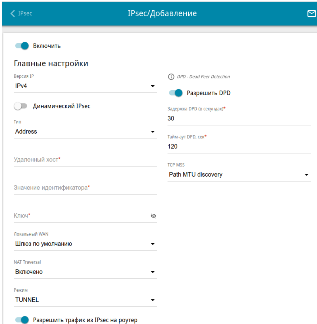
Рисунок 158. Страница добавления IPsec-туннеля. Раздел Главные настройки .
