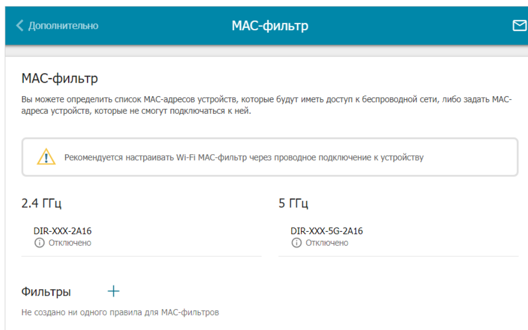
Рисунок 118. Страница для настройки MAC-фильтра для беспроводной сети.
