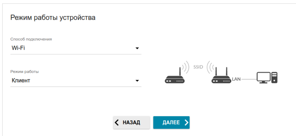
Рисунок 38. Выбор режима работы устройства. Режим Клиент .
