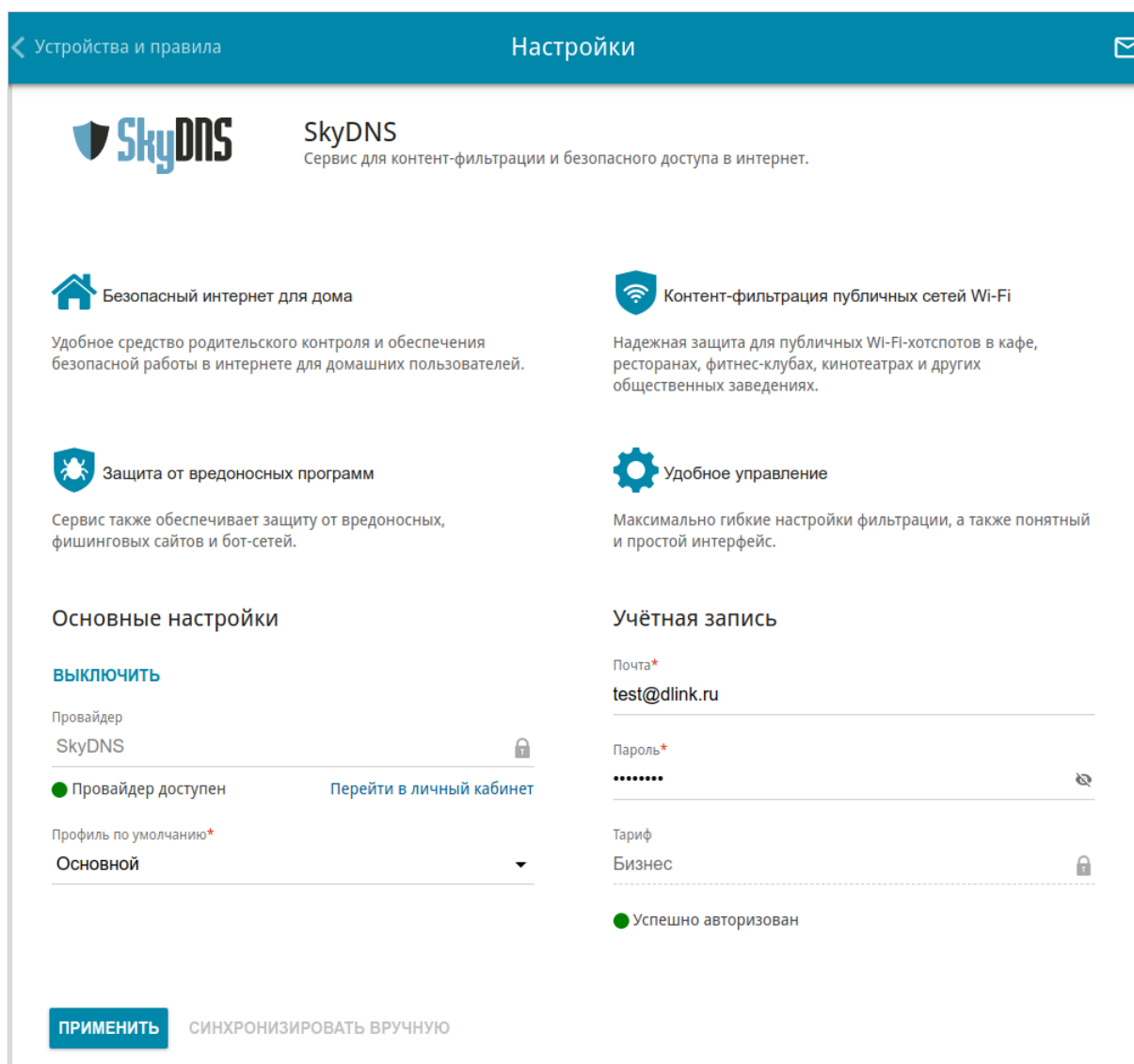
Рисунок 187. Страница SkyDNS / Настройки .
