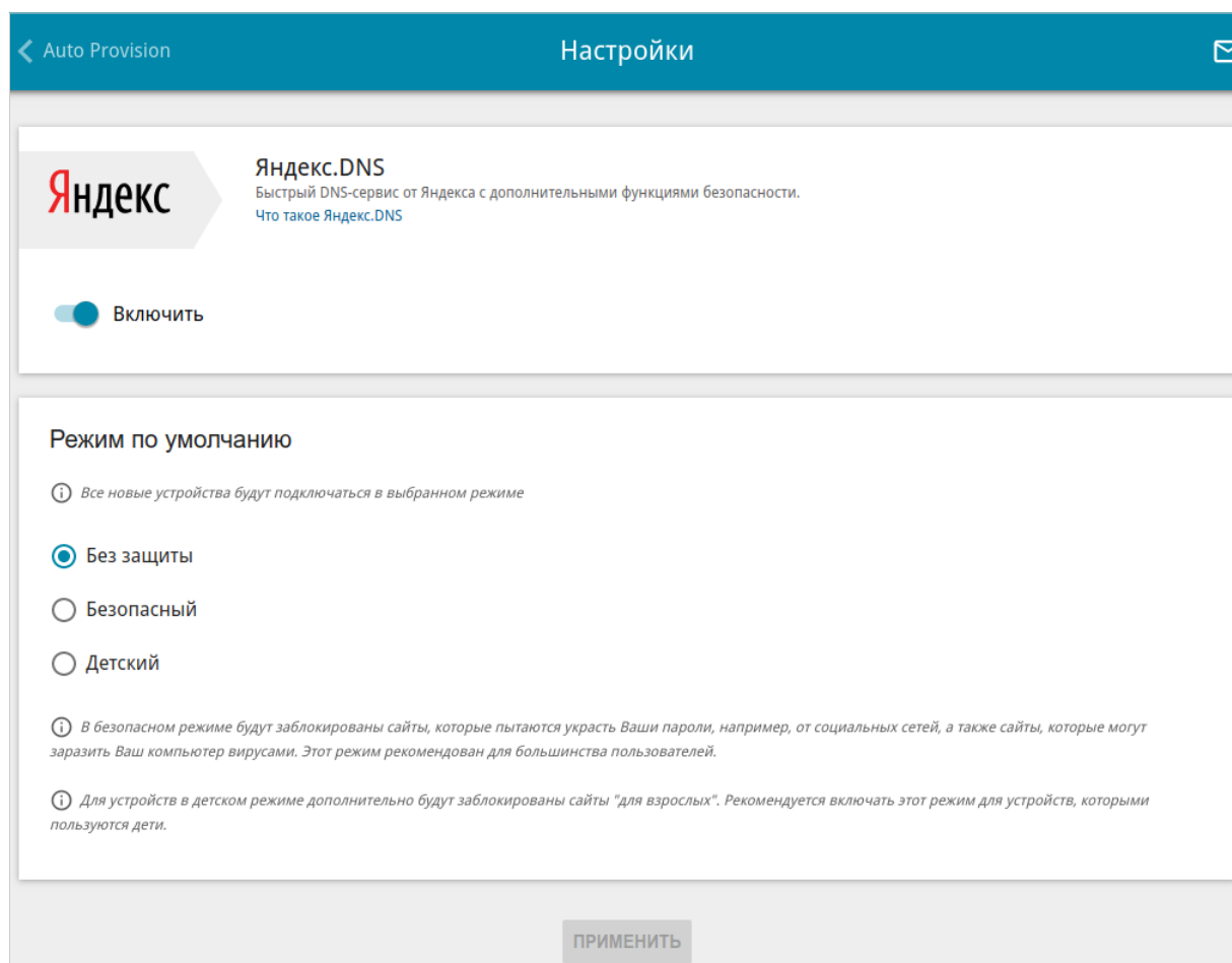
Рисунок 184. Страница Яндекс.DNS / Настройки .
