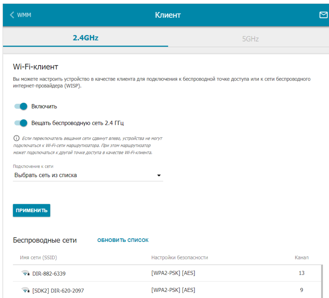
Рисунок 114. Страница для настройки маршрутизатора в качестве клиента.
