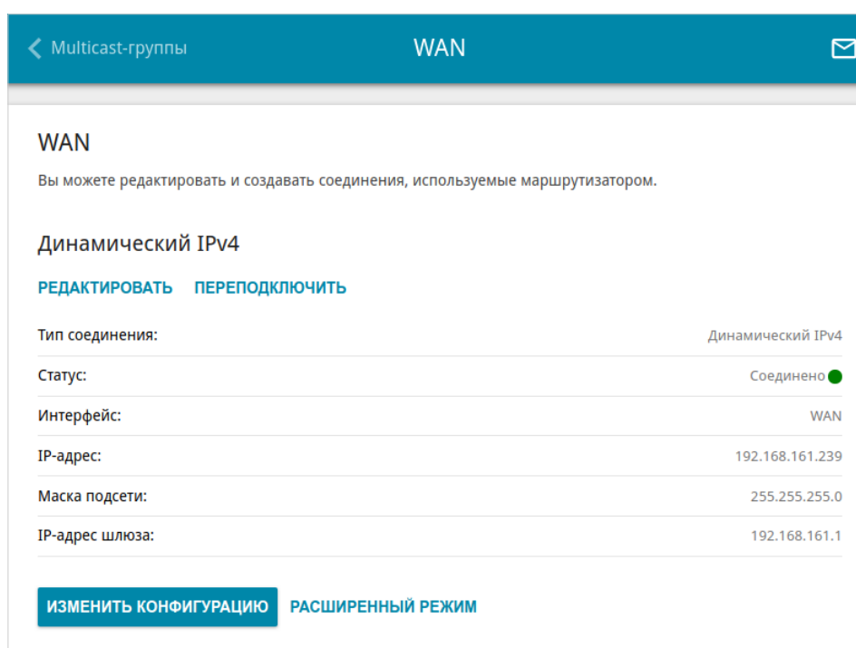
Рисунок 65. Страница Настройка соединений / WAN . Упрощенный режим.
