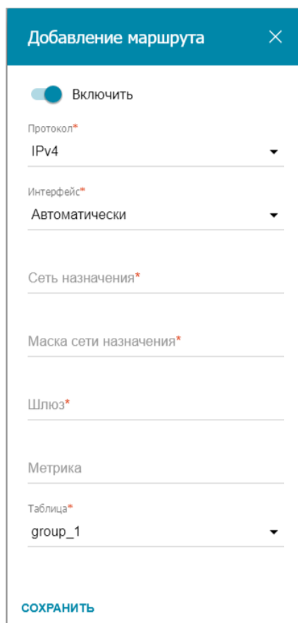
Рисунок 150. Окно добавления нового маршрута.
