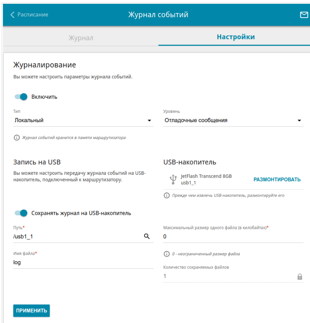
Рисунок 175. Страница Система / Журнал событий . Вкладка Настройки .
