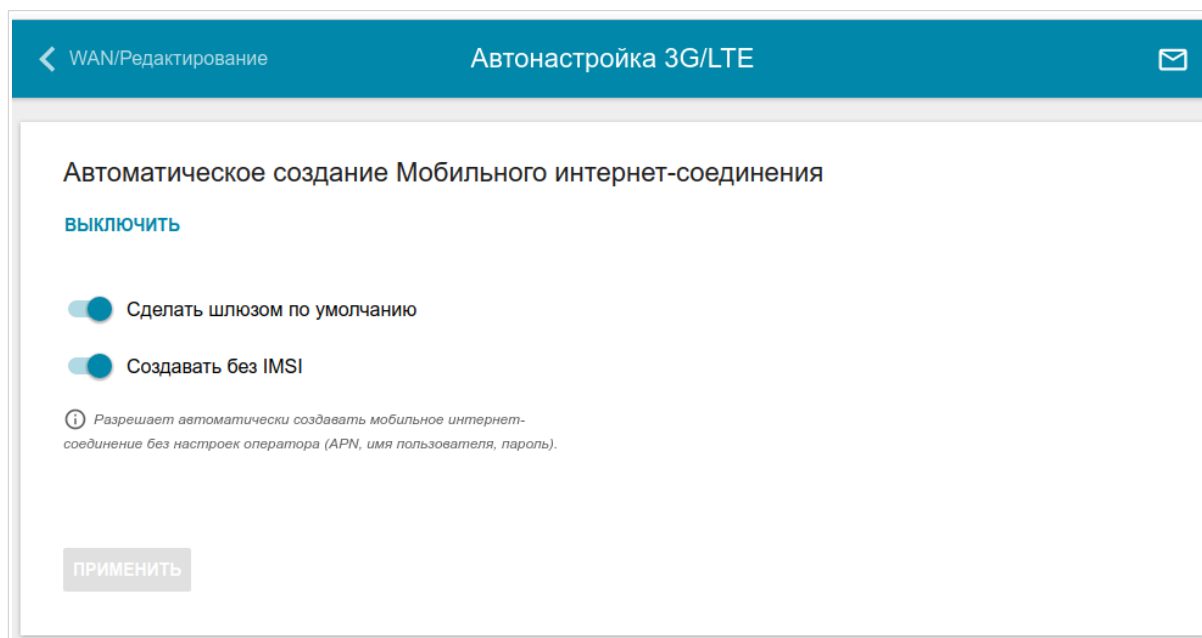
Рисунок 103. Страница Настройка соединений / Автонастройка 3G/LTE .
