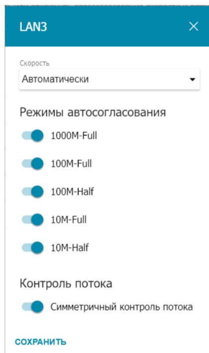
Рисунок 147. Окно изменения настроек порта маршрутизатора.
