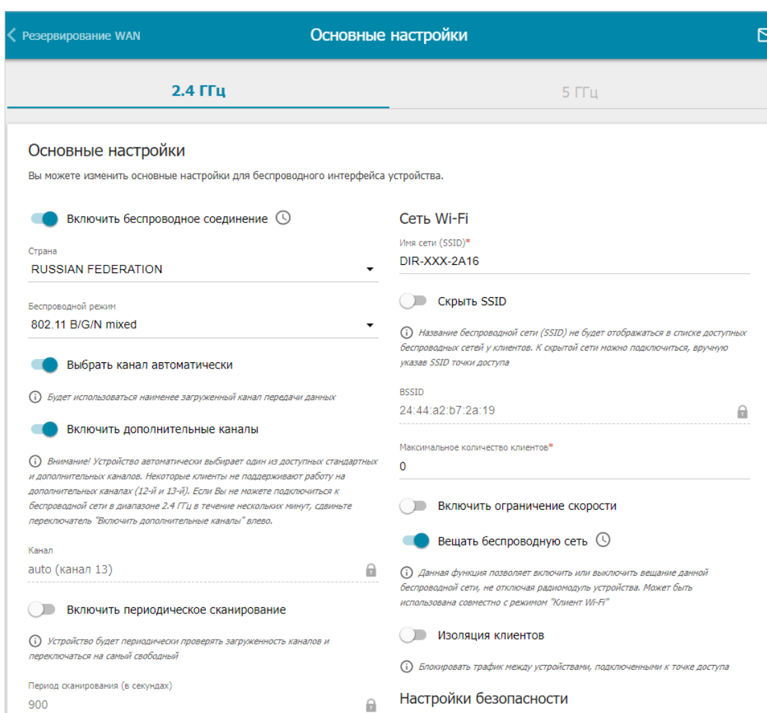
Рисунок 104. Основные настройки беспроводной локальной сети в диапазоне 2,4 ГГц.
