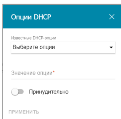
Рисунок 93. Настройка локального интерфейса. Вкладка IPv4 . Окно для настройки опции DHCP.
