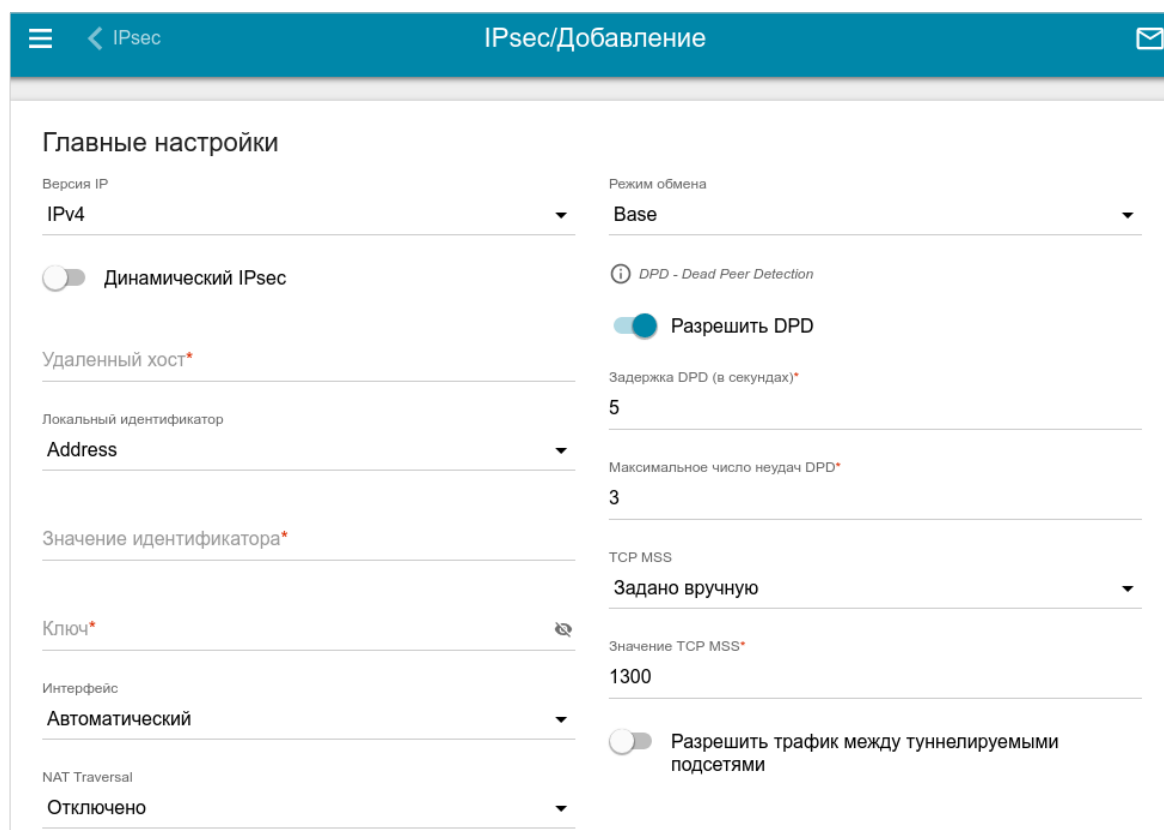
Рисунок 156. Страница добавления IPsec-туннеля. Раздел Основные настройки .
