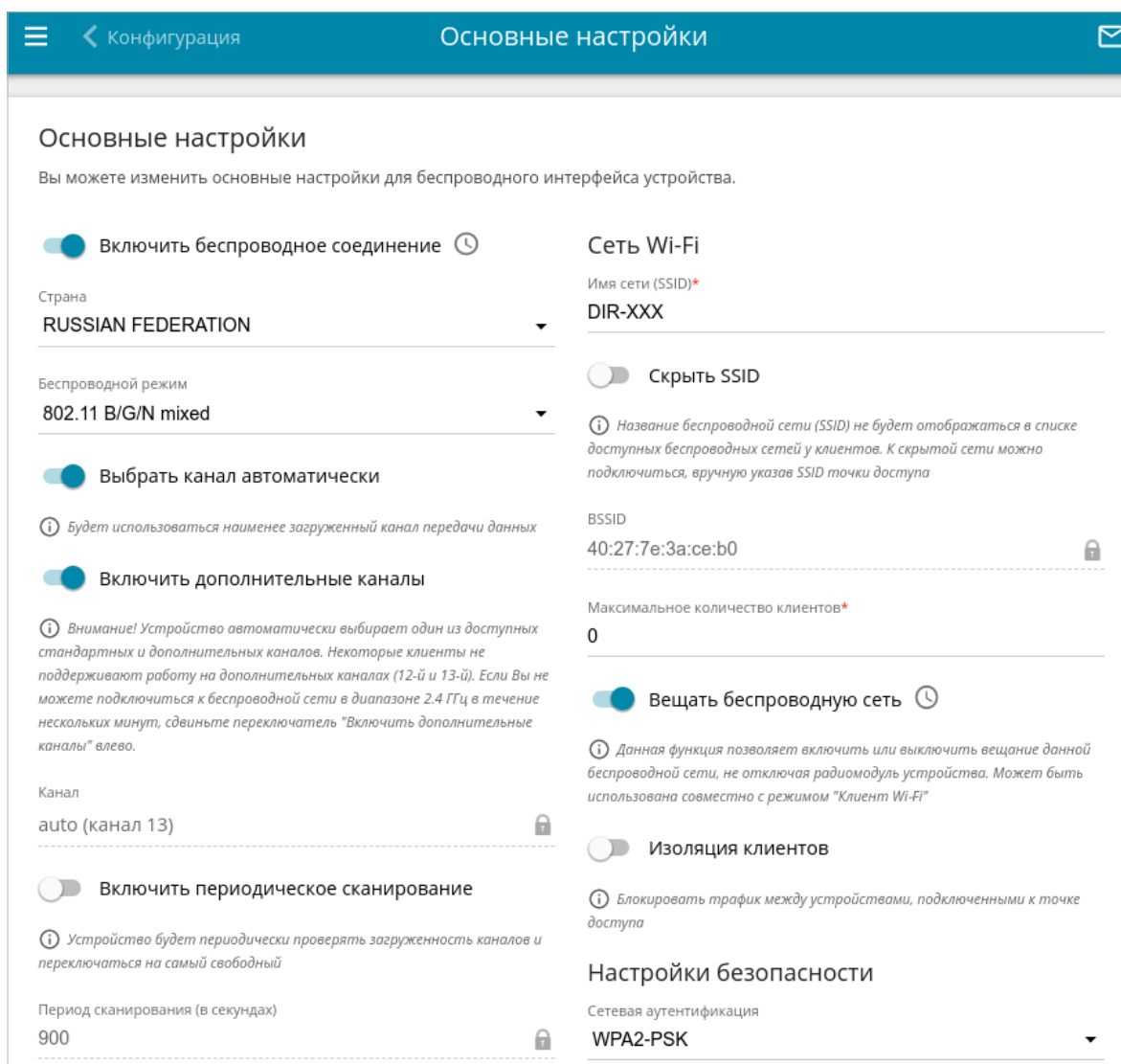
Рисунок 103. Общие настройки беспроводного соединения.
