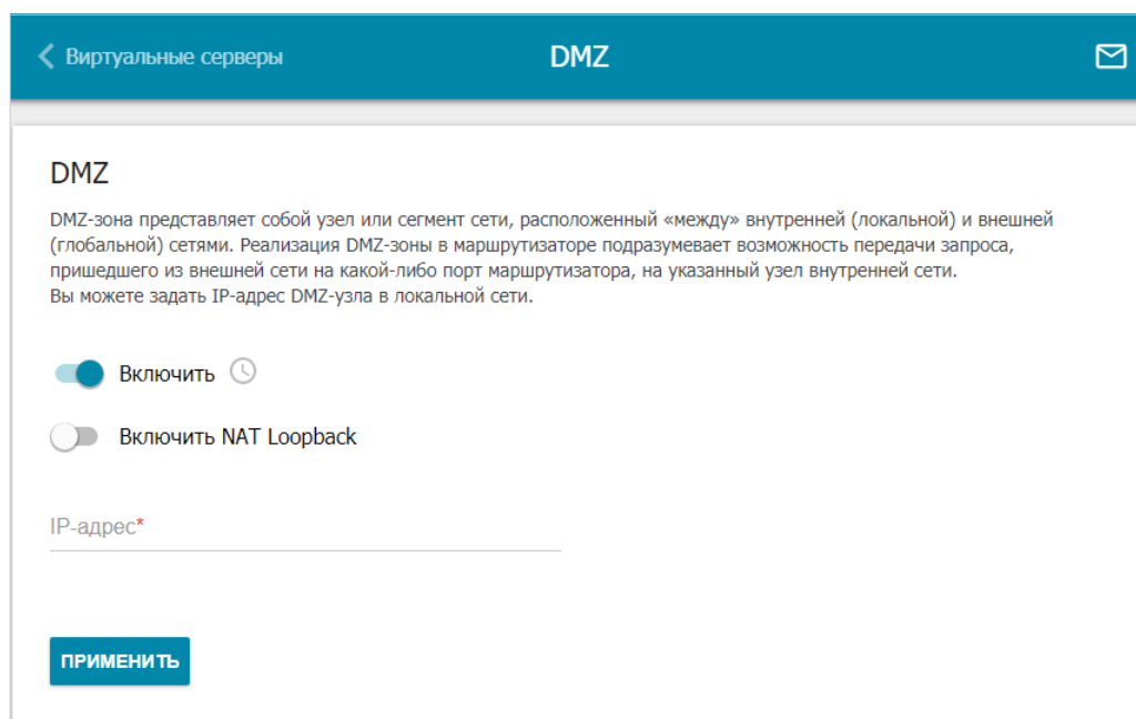
Рисунок 163. Страница Межсетевой экран / DMZ .
