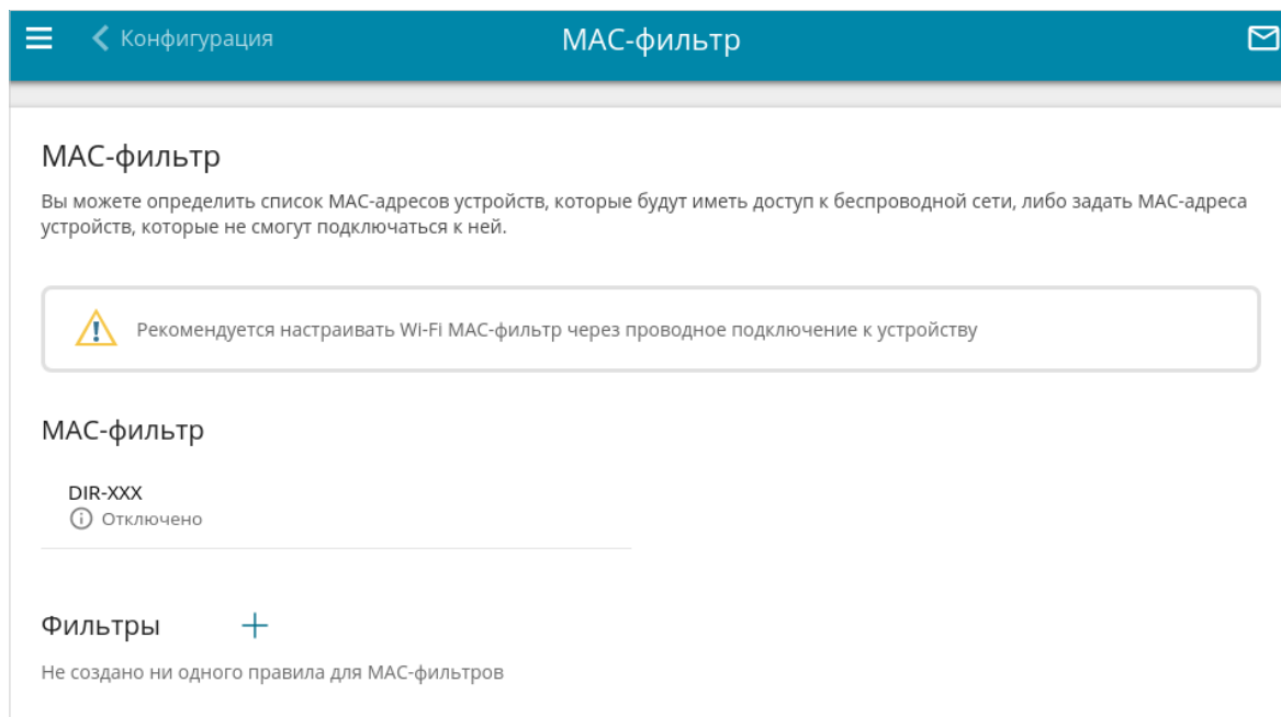
Рисунок 115. Страница для настройки MAC-фильтра для беспроводной сети.
