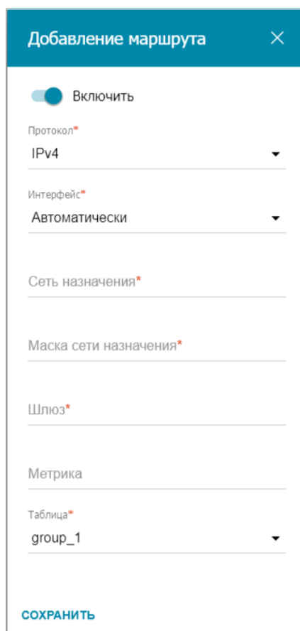
Рисунок 152. Окно добавления нового маршрута.
