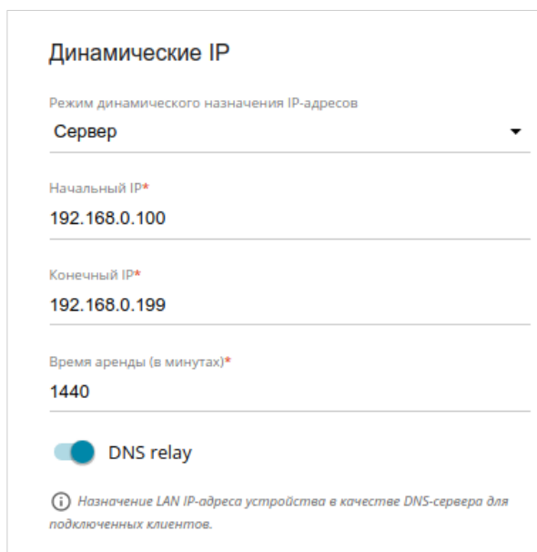
Рисунок 90. Настройка локального интерфейса. Вкладка IPv4. Раздел Динамические IP.
