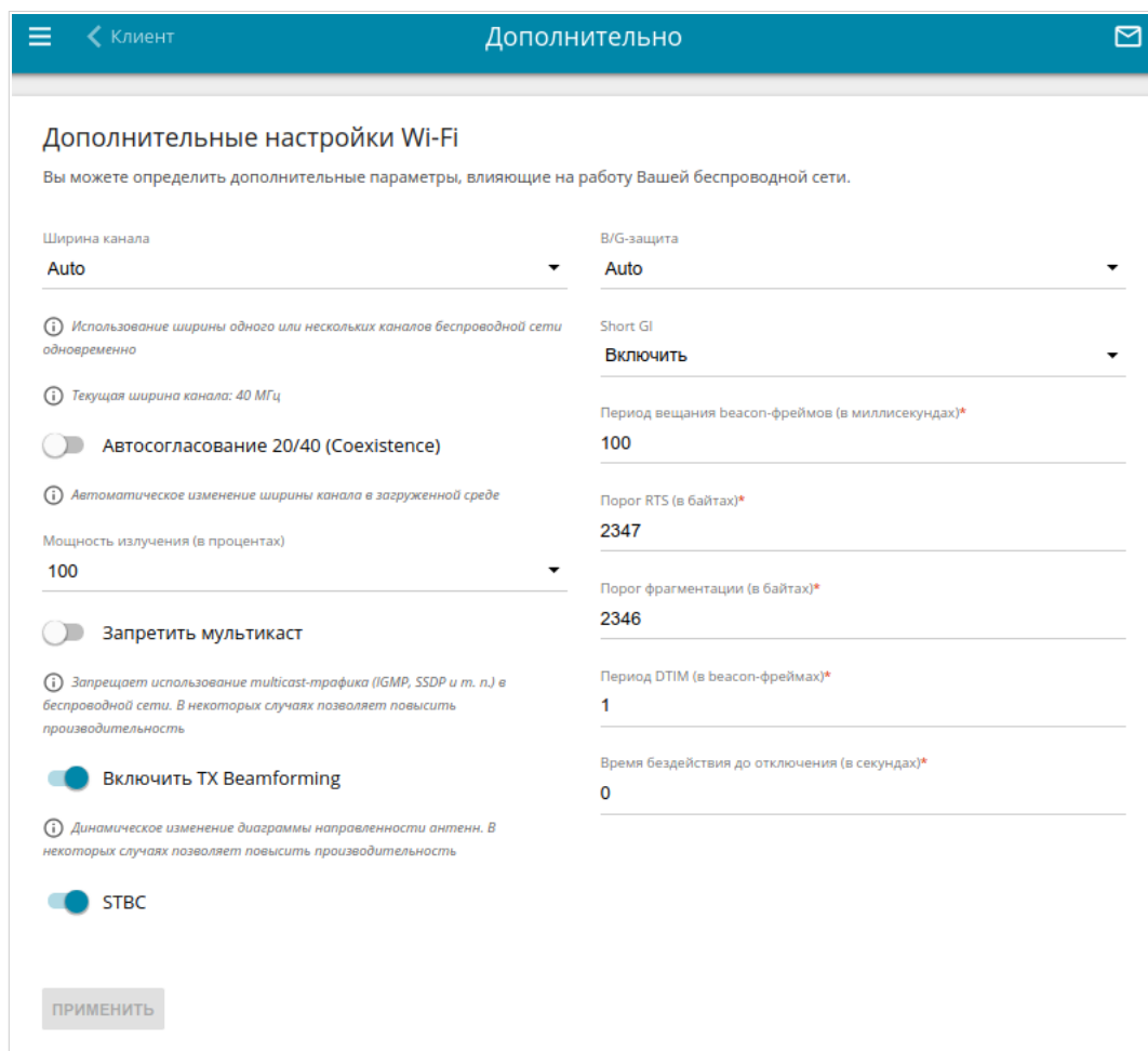
Рисунок 114. Страница дополнительных настроек для беспроводной сети.
