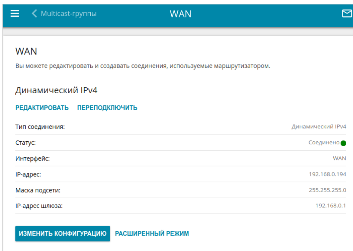
Рисунок 65. Страница Настройка соединений / WAN . Упрощенный режим.
