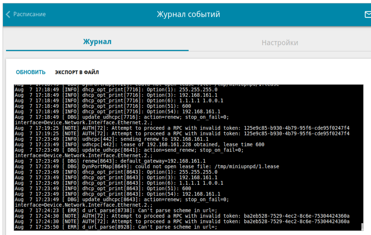
Рисунок 175. Страница Система / Журнал событий . Вкладка Журнал .
