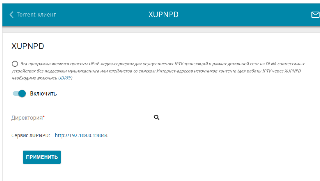
Рисунок 130. Страница USB-накопитель / XUPNPD .
