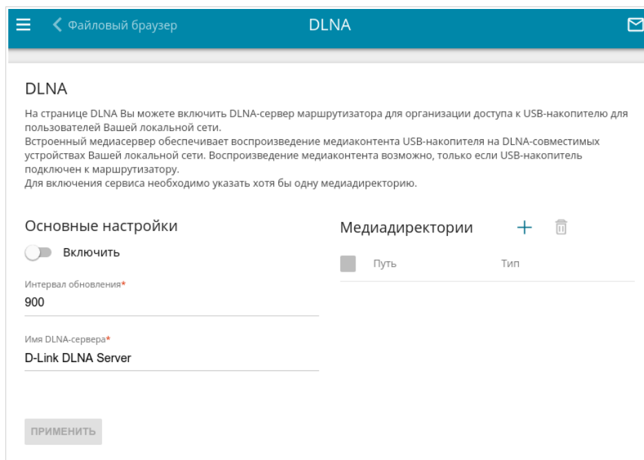
Рисунок 126. Страница USB-накопитель / DLNA .
