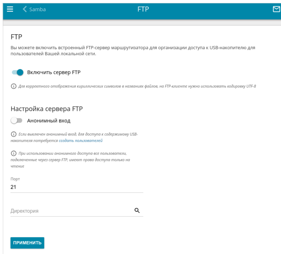
Рисунок 124. Страница USB-накопитель / FTP .
