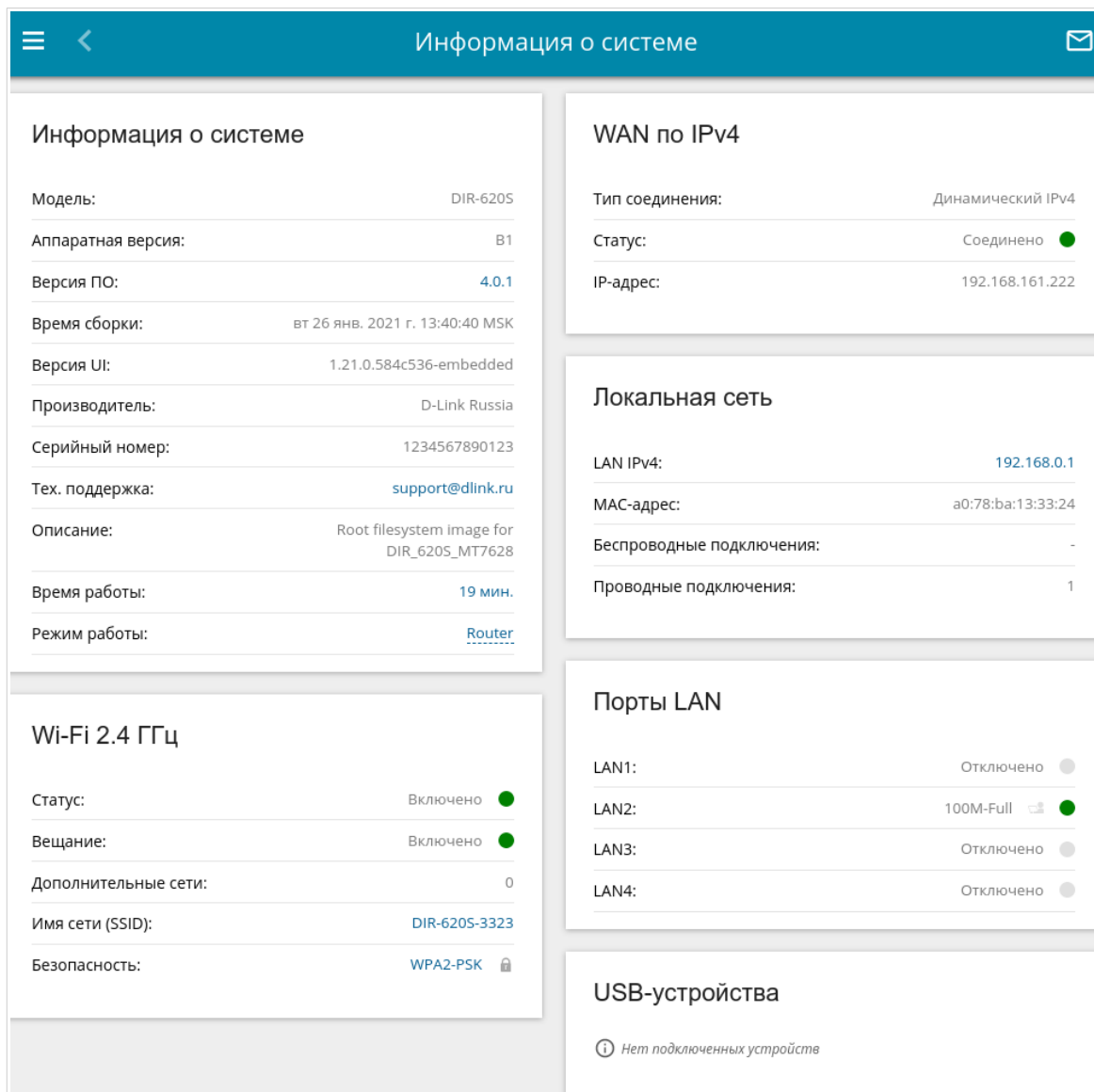
Рисунок 26. Страница информации о системе.
