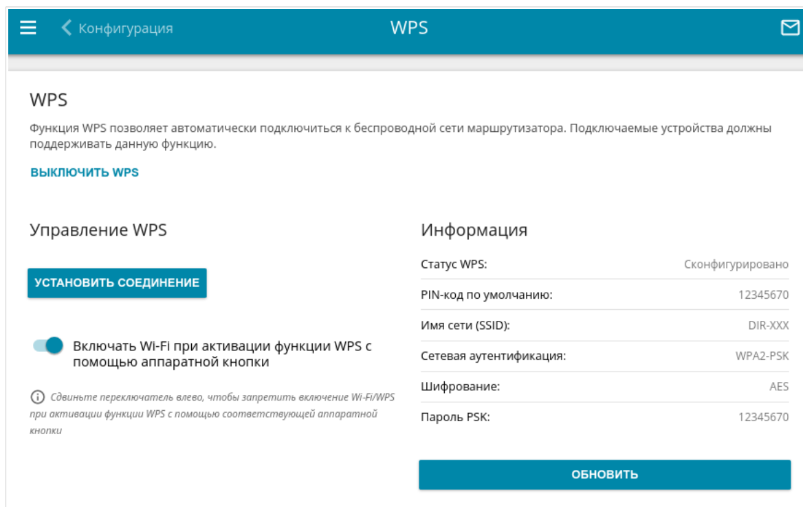
Рисунок 110. Страница для настройки функции WPS.
