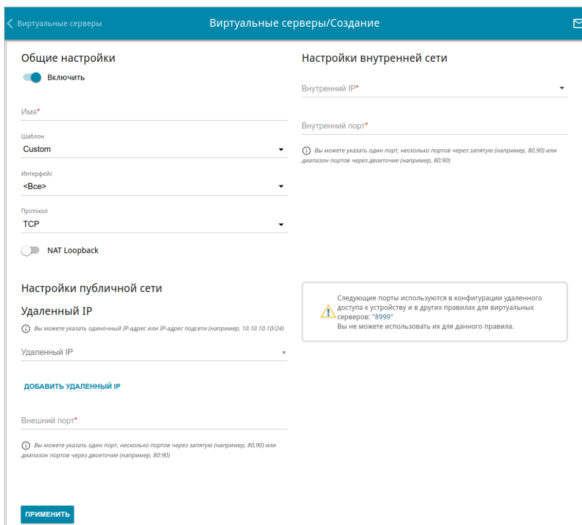
Рисунок 162. Страница добавления виртуального сервера.
