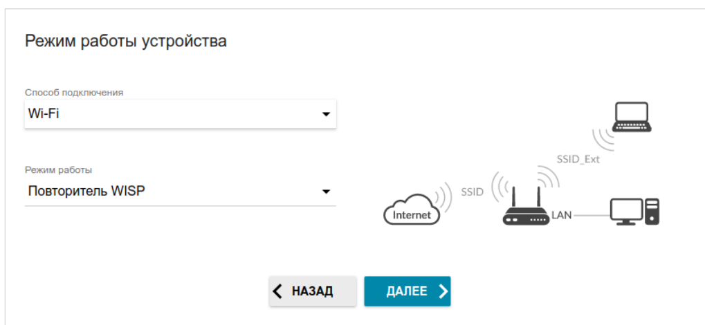
Рисунок 36. Выбор режима работы устройства. Режим Повторитель WISP .
