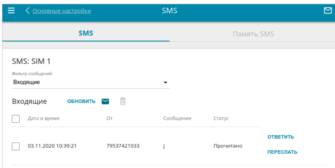
Рисунок 136. Страница USB-модем / Название модема / SMS . Вкладка SMS .
