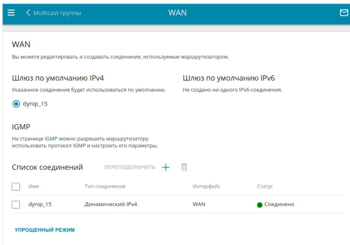
Рисунок 66. Страница Настройка соединений / WAN . Расширенный режим.
