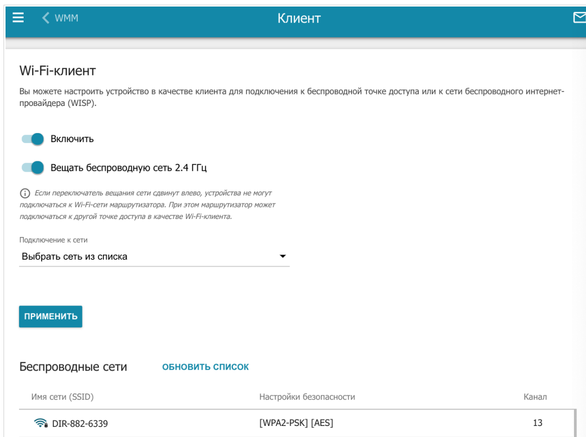
Рисунок 113. Страница для настройки маршрутизатора в качестве клиента.
