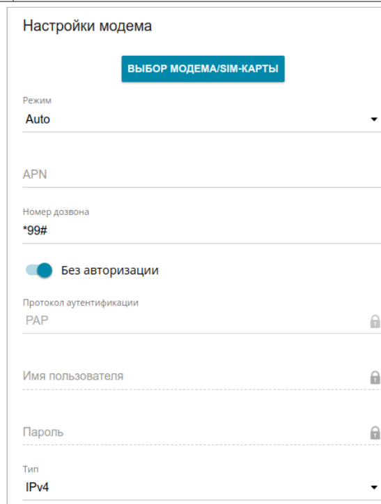
Рисунок 86. Страница добавления соединения типа Мобильный интернет . Раздел Настройки модема .
