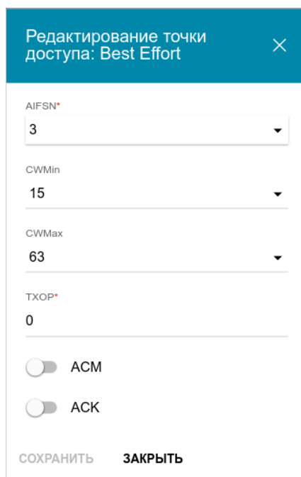
Рисунок 112. Окно для изменения параметров функции WMM.
