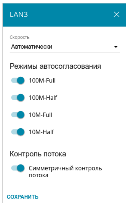
Рисунок 149. Окно изменения настроек порта маршрутизатора.
