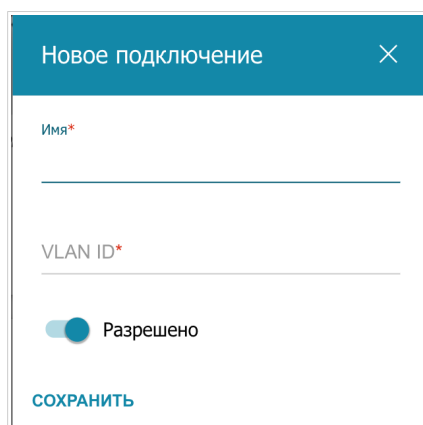
Рисунок 58. Добавление подключения.
