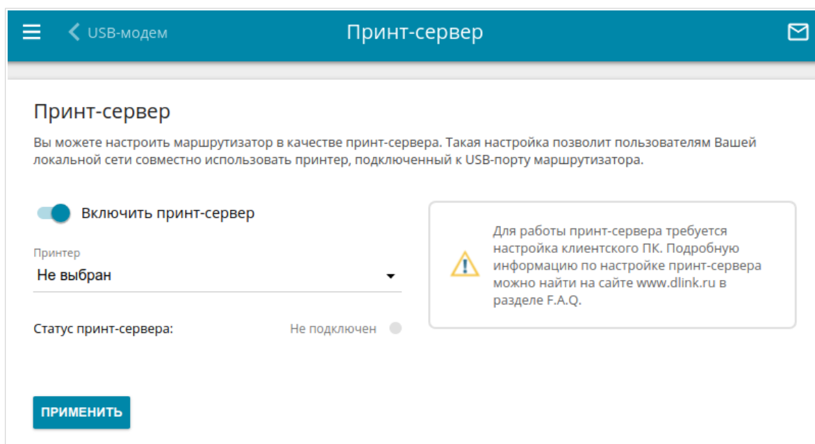
Рисунок 118. Страница Принт-сервер .
