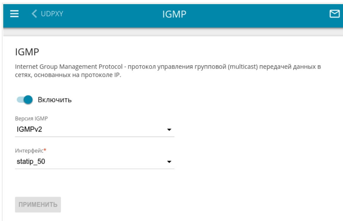
Рисунок 157. Страница Дополнительно / IGMP .
