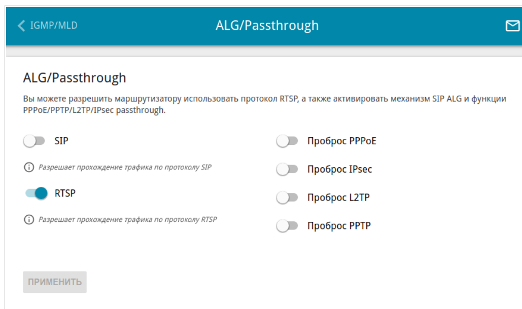
Рисунок 158. Страница Дополнительно / ALG/Passthrough .
