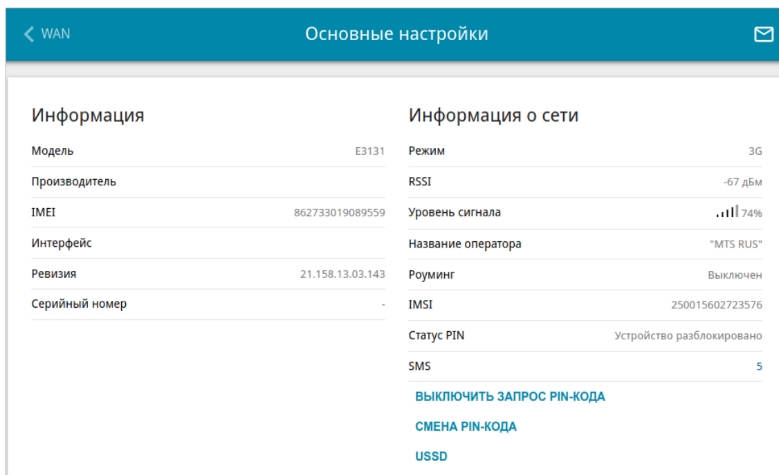
Рисунок 134. Страница USB-модем / Название модема / Основные настройки .
