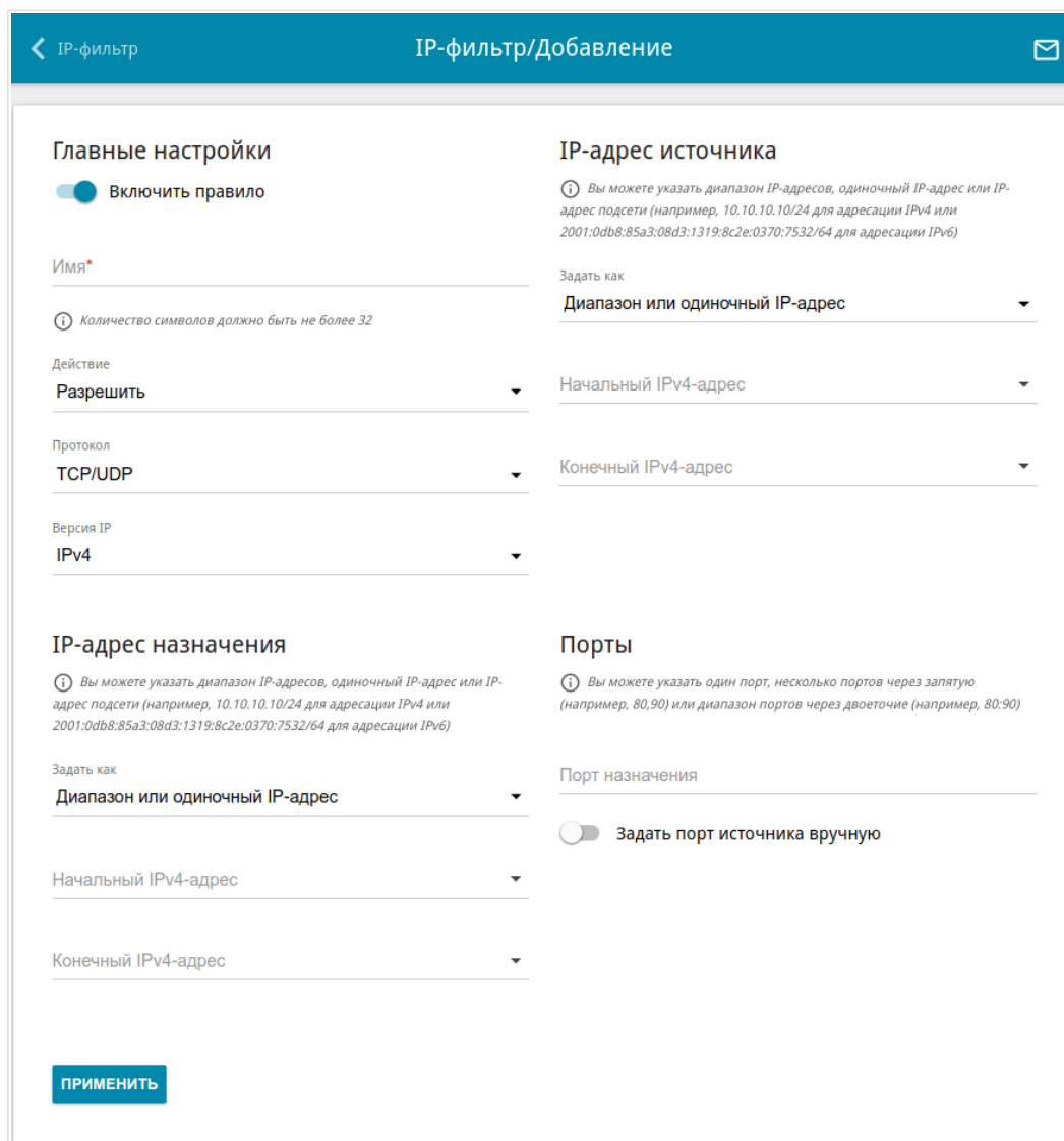
Рисунок 126. Страница добавления правила для обработки сетевых пакетов.
