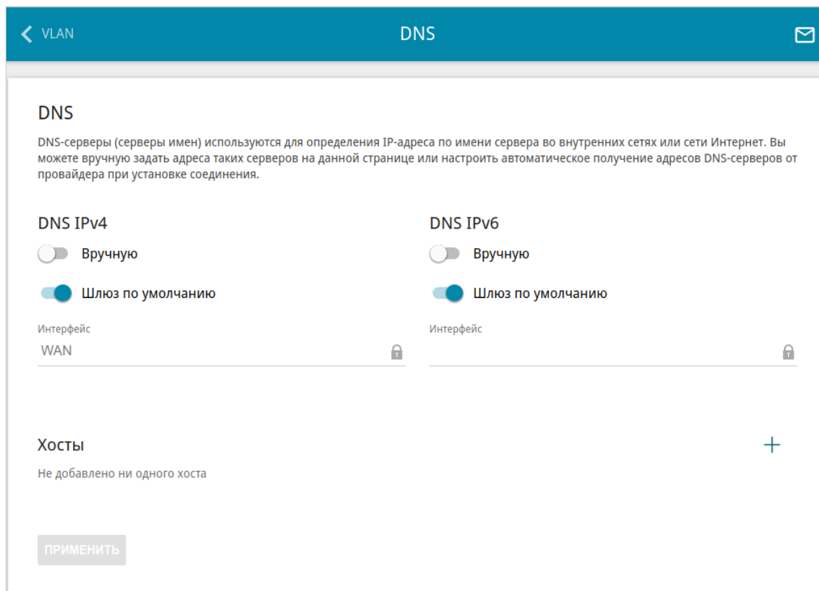
Рисунок 102. Страница Дополнительно / DNS .
