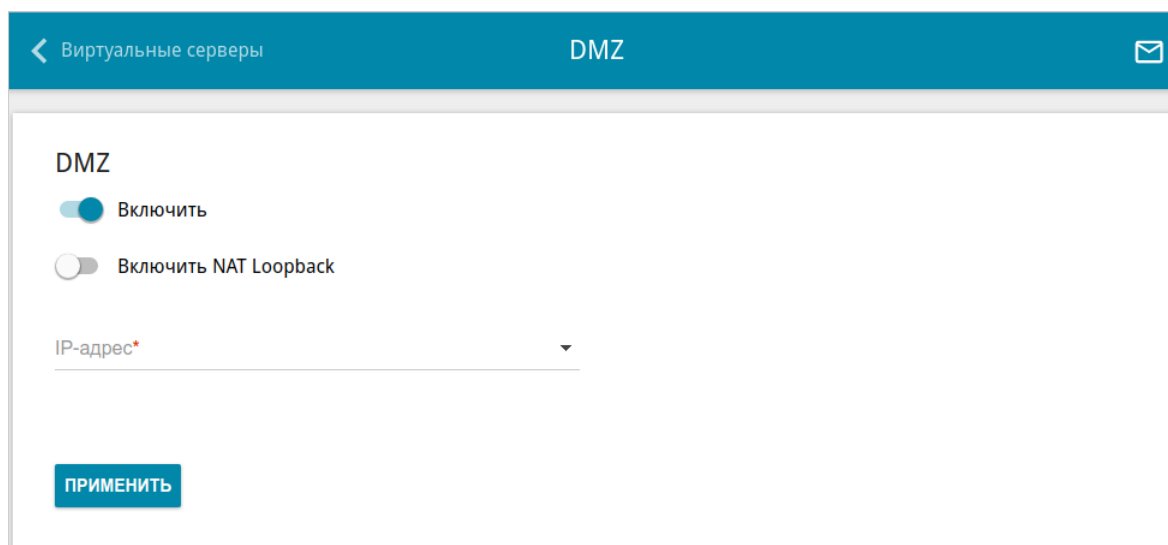
Рисунок 129. Страница Межсетевой экран / DMZ .
