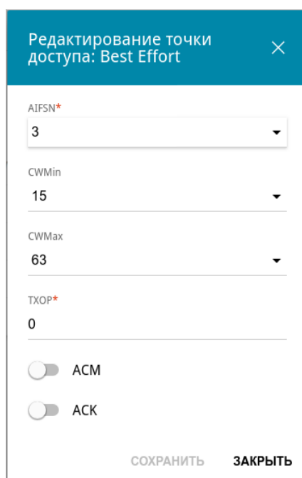
Рисунок 92. Окно для изменения параметров функции WMM.
