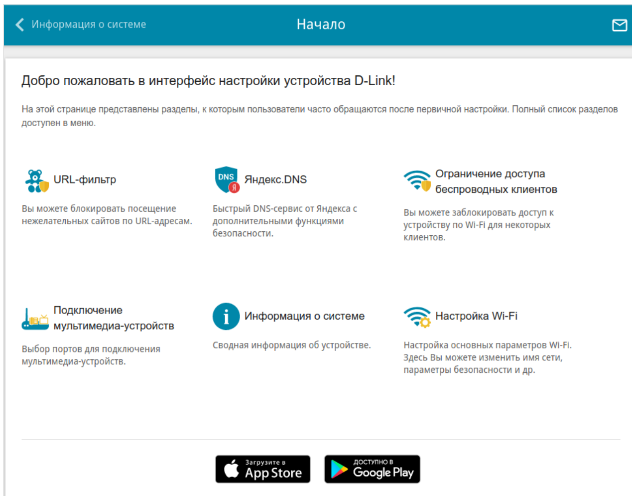
Рисунок 16. Страница Начало .
