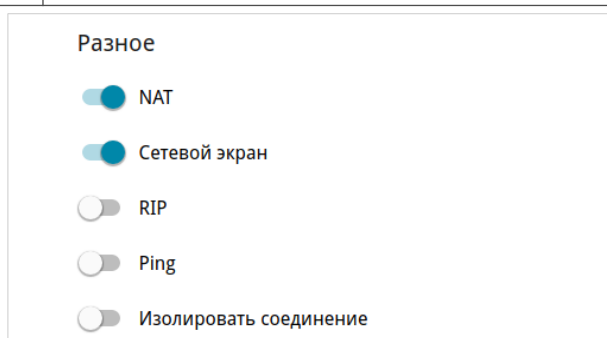
Рисунок 65. Страница добавления соединения типа PPPoE . Раздел Разное .
