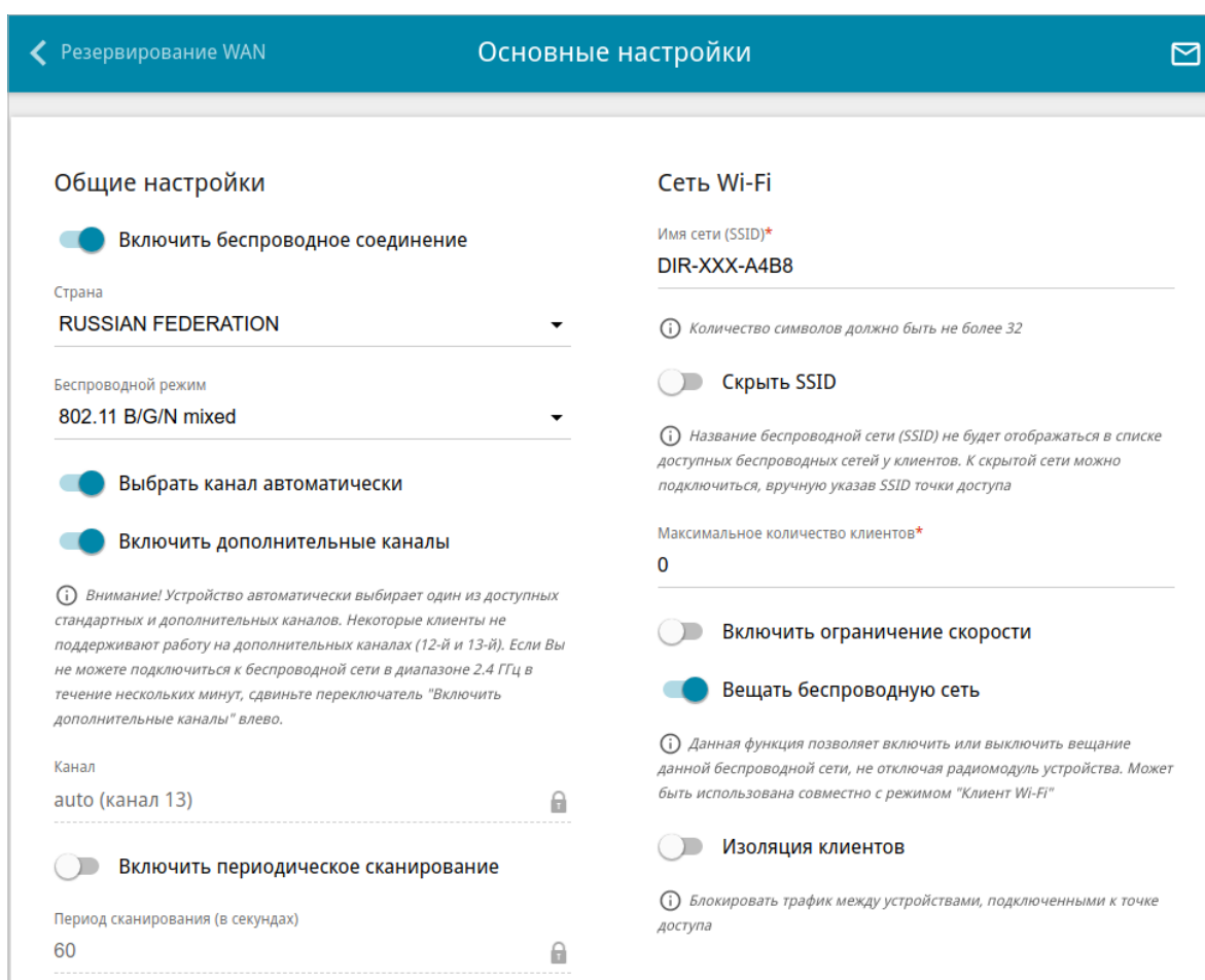
Рисунок 83. Общие настройки беспроводного соединения.
