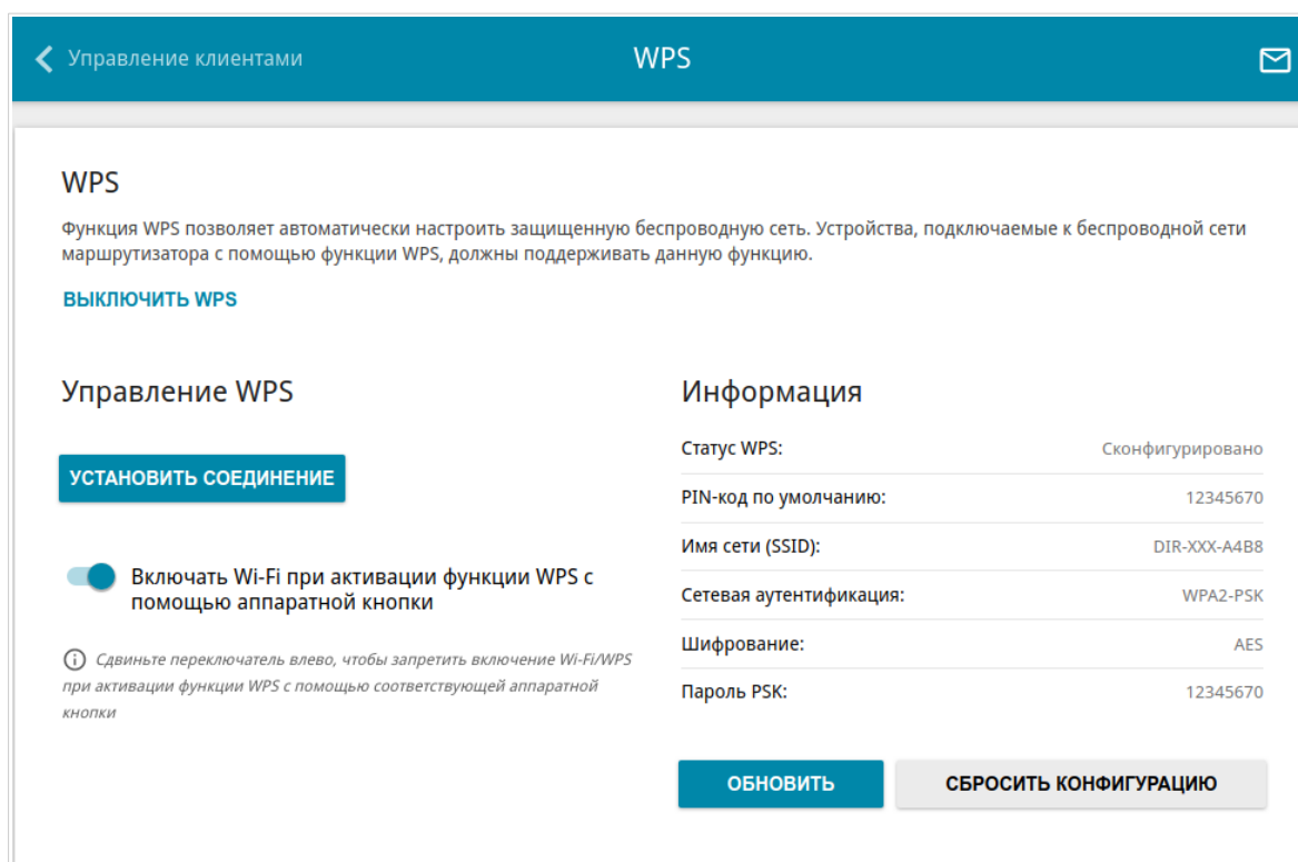
Рисунок 90. Страница для настройки функции WPS.
