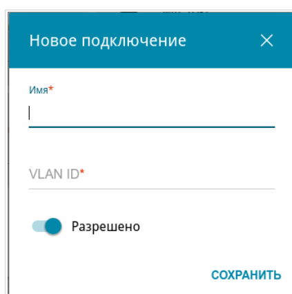
Рисунок 44. Добавление подключения.
