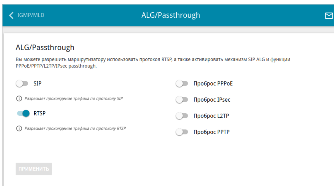
Рисунок 120. Страница Дополнительно / ALG/Passthrough .
