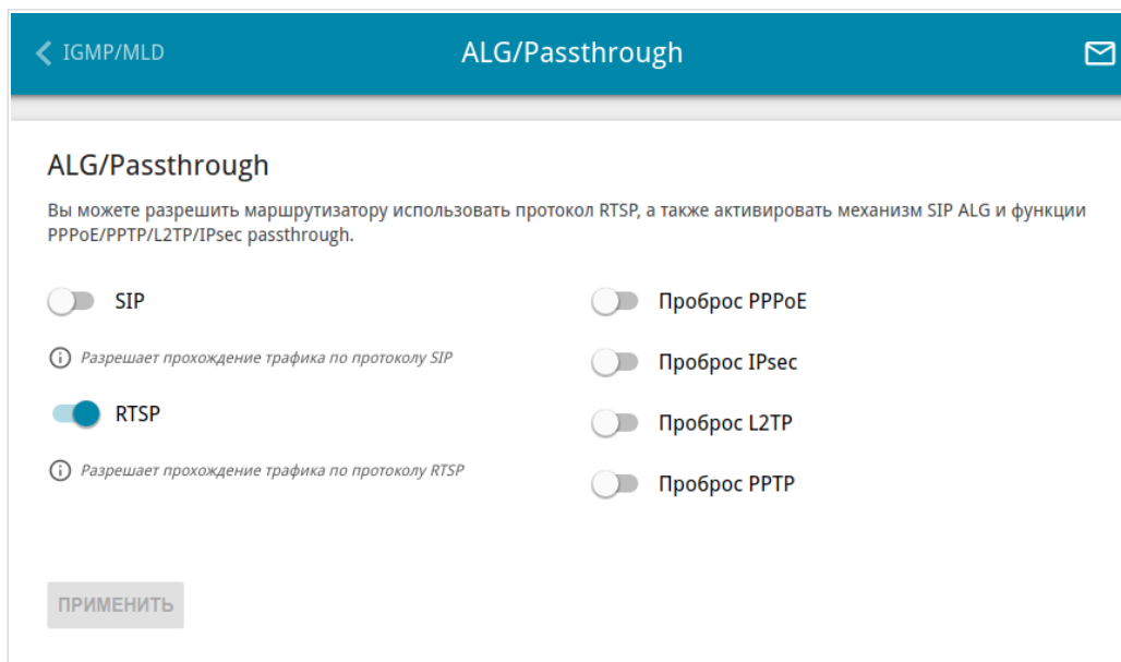
Рисунок 128. Страница Дополнительно / ALG/Passthrough .
