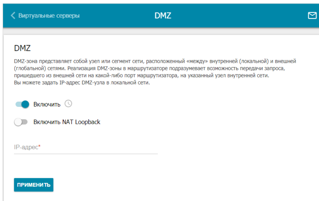
Рисунок 133. Страница Межсетевой экран / DMZ .
