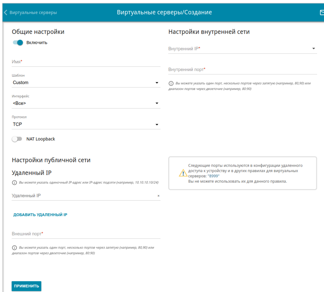
Рисунок 132. Страница добавления виртуального сервера.
