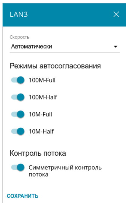
Рисунок 119. Окно изменения настроек порта маршрутизатора.
