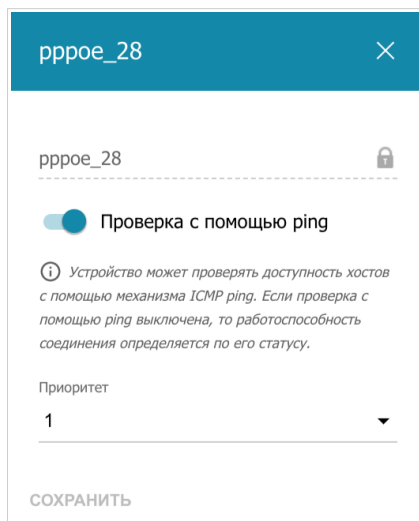
Рисунок 94. Окно изменения уровня приоритета соединения.
