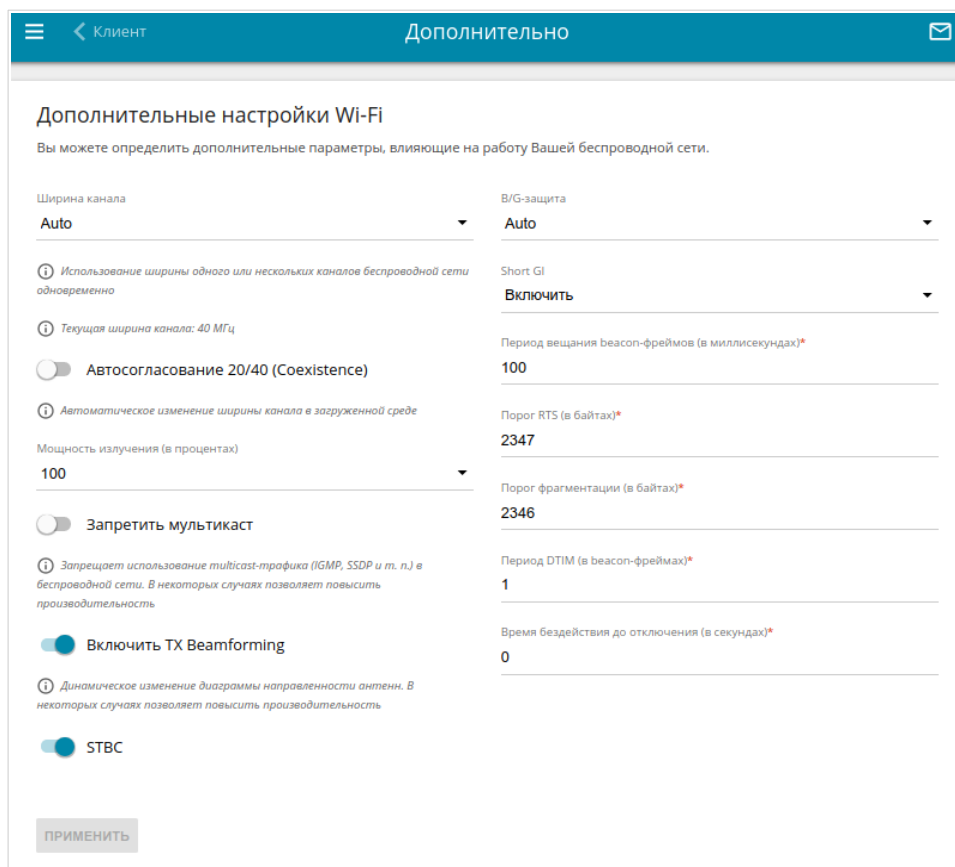
Рисунок 106. Страница дополнительных настроек для беспроводной сети.
