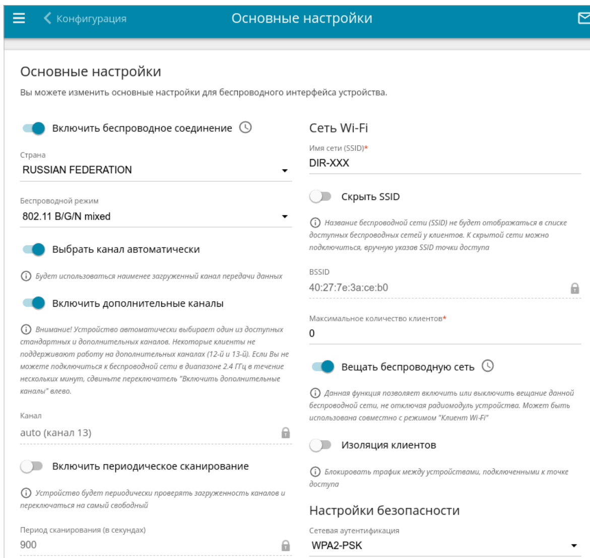
Рисунок 95. Общие настройки беспроводного соединения.
