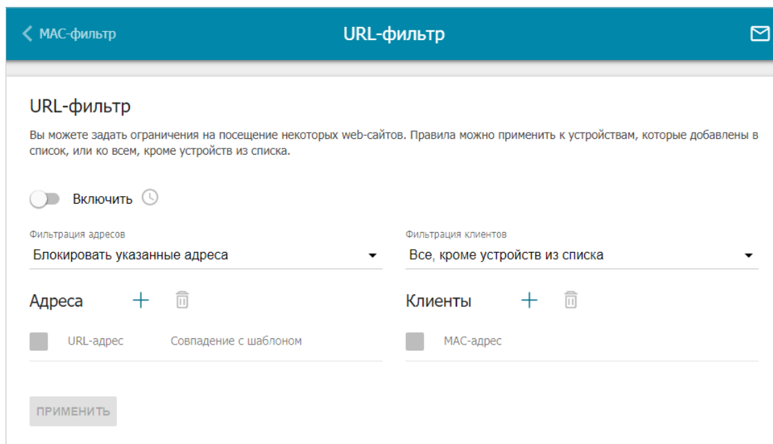
Рисунок 136. Страница Межсетевой экран / URL-фильтр .
