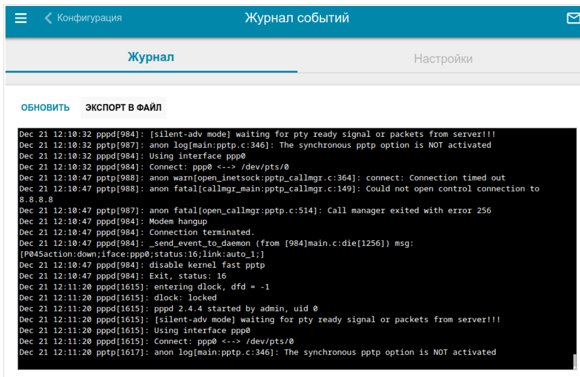
Рисунок 145. Страница Система / Журнал событий. Вкладка Журнал.
