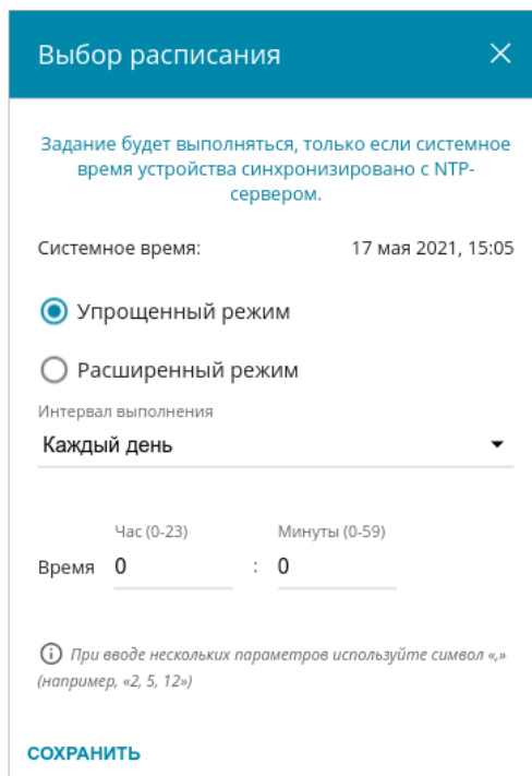
Рисунок 142. Окно настройки автоматической перезагрузки устройства по расписанию.
