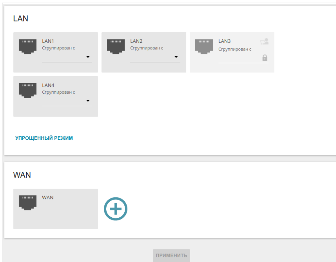
Рисунок 54. Мастер подключения мультимедиа-устройств. Расширенный режим.
