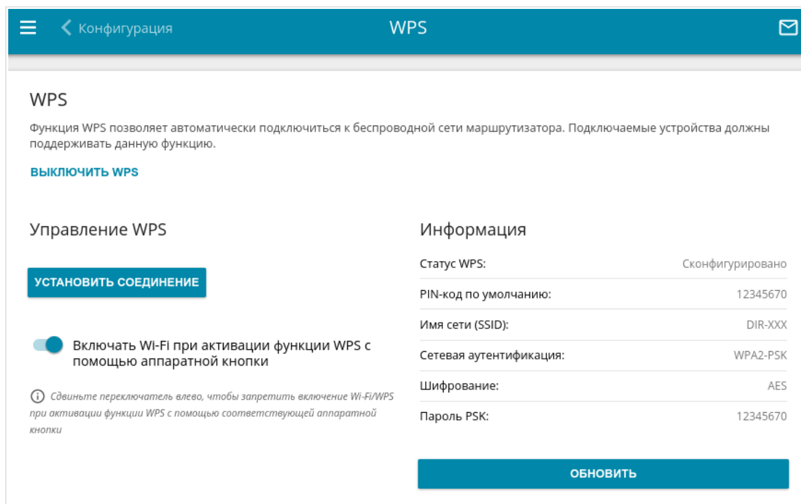
Рисунок 102. Страница для настройки функции WPS.
