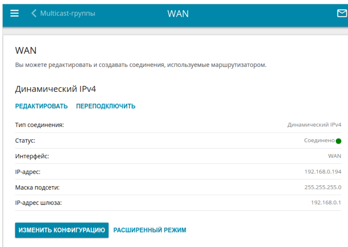
Рисунок 62. Страница Настройка соединений / WAN . Упрощенный режим.
