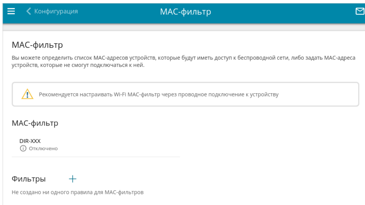
Рисунок 107. Страница для настройки MAC-фильтра для беспроводной сети.
