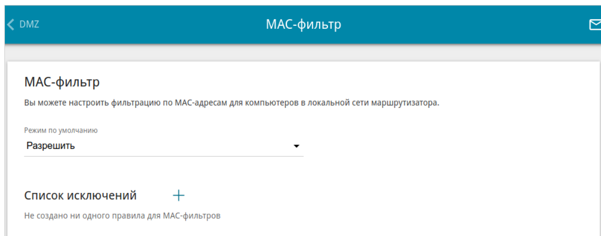
Рисунок 134. Страница Межсетевой экран / MAC-фильтр .
