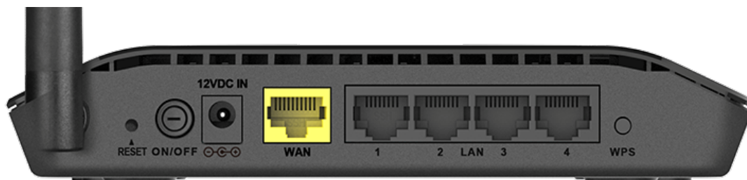
Рисунок 2. Вид задней панели DIR-300S.
