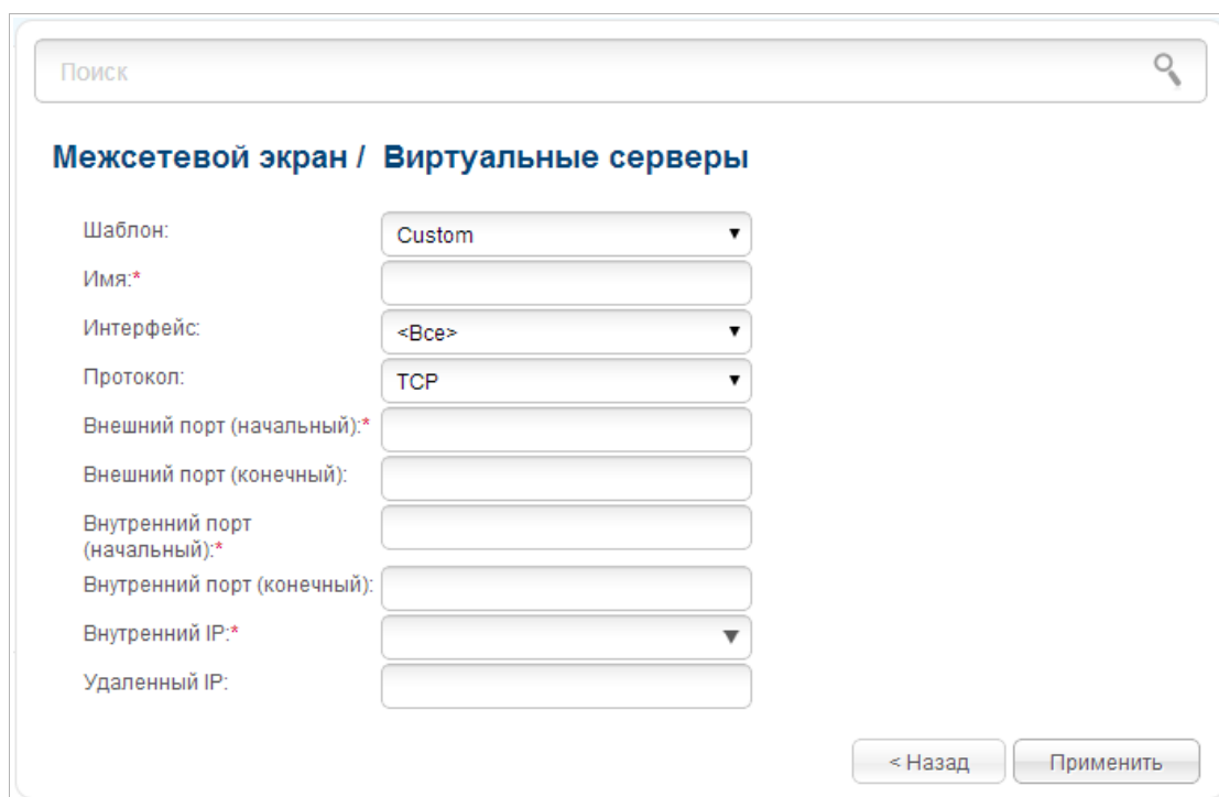
Рисунок 150. Страница добавления виртуального сервера.
