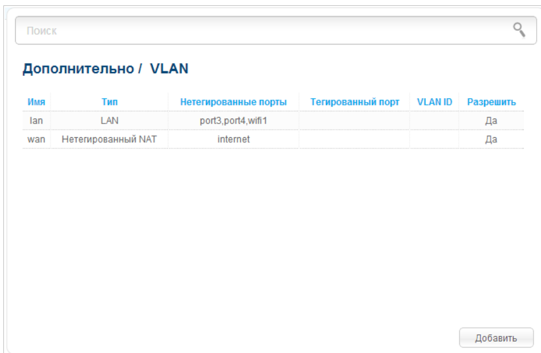
Рисунок 137. Страница Дополнительно / VLAN .
