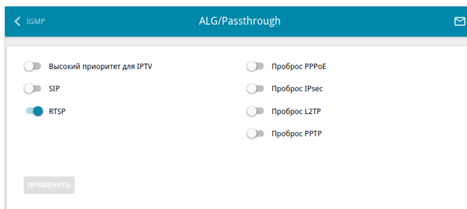
Рисунок 120. Страница Дополнительно / ALG/Passthrough .
