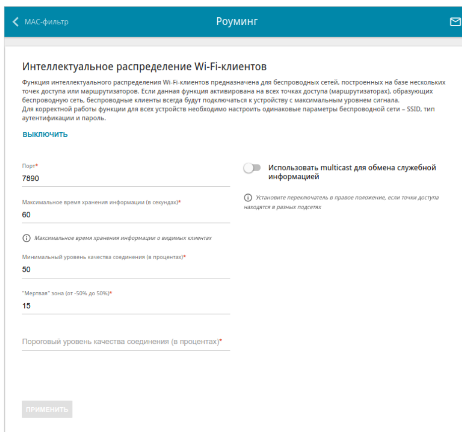
Рисунок 99. Страница Wi-Fi / Роуминг .
