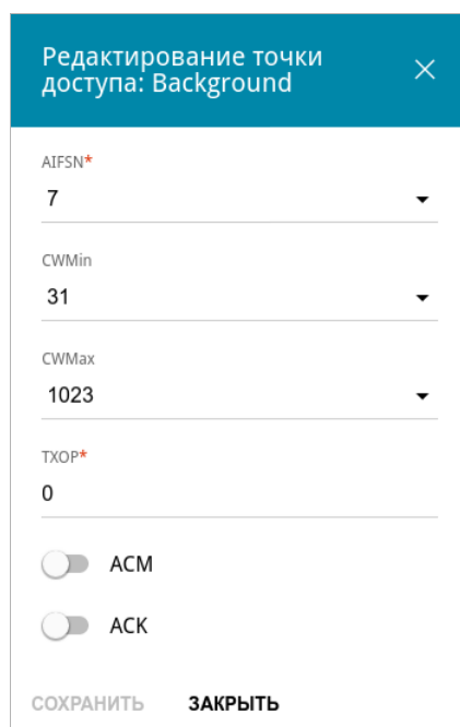
Рисунок 139. Окно для изменения параметров функции WMM.
