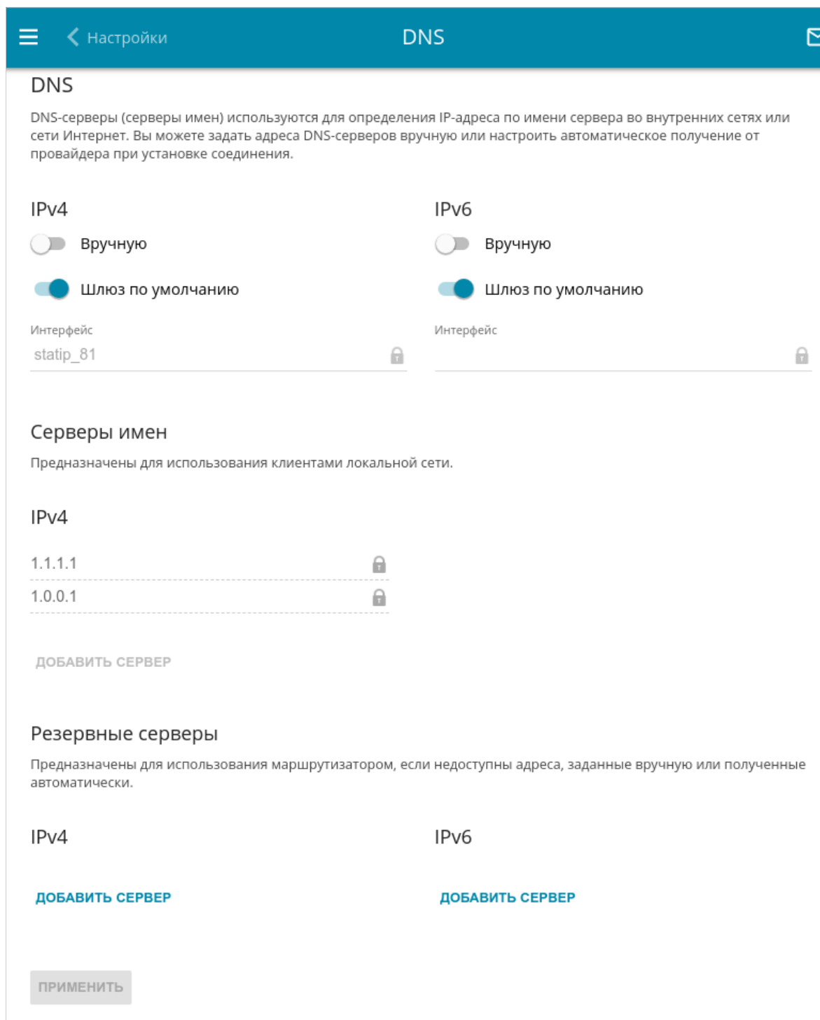
Рисунок 172. Страница Дополнительно / DNS .
